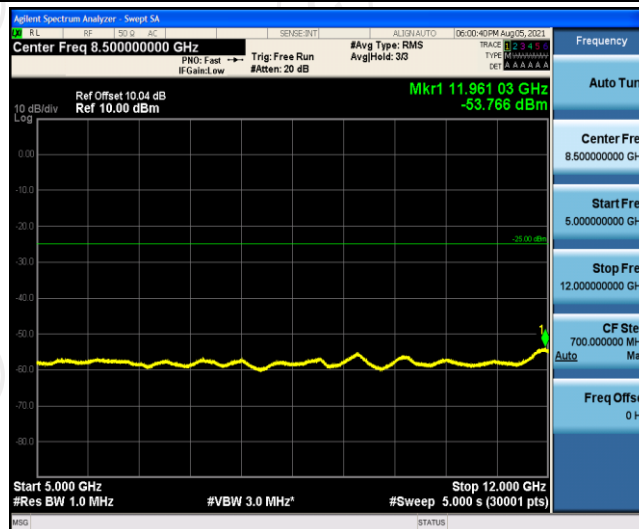
Band7-10MHz-QPSK-20800-1RB#0-Range6:12000~26500MHz
