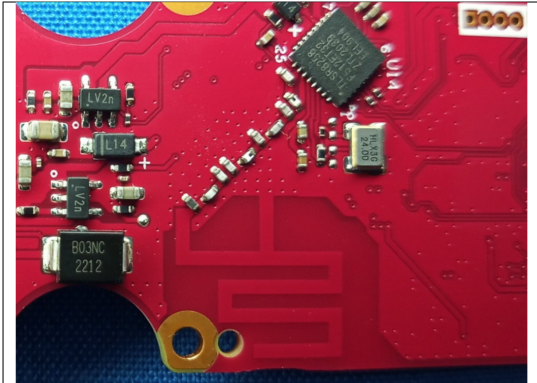
BLE Chip
