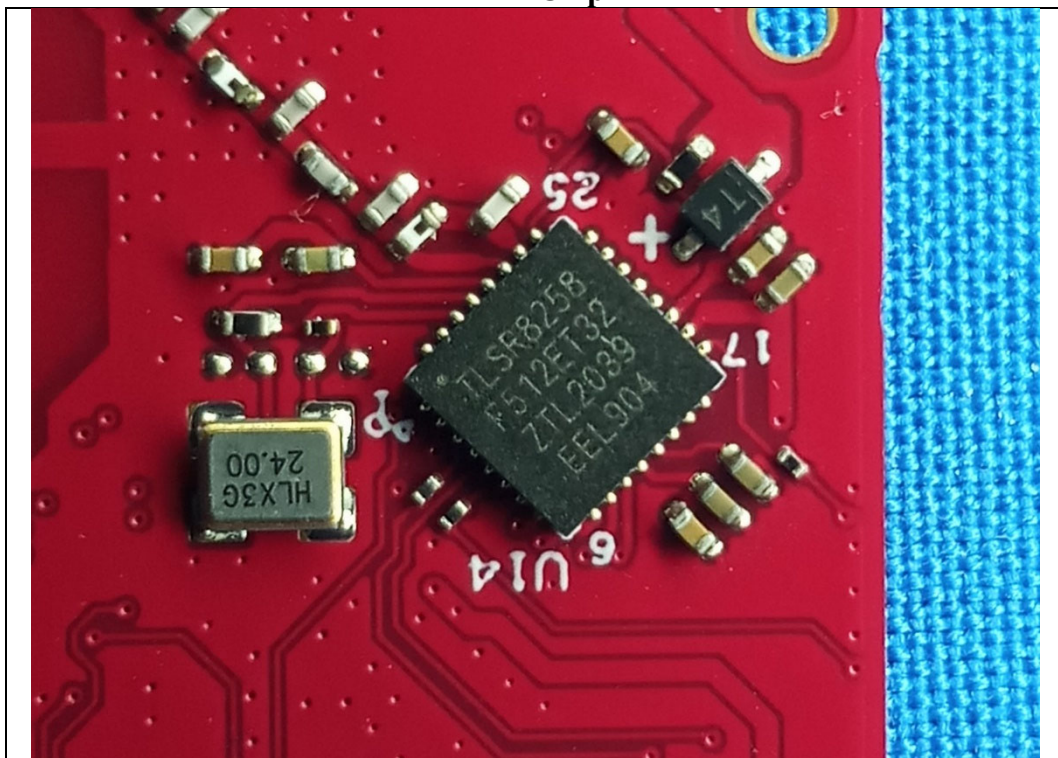
BLE Chip
