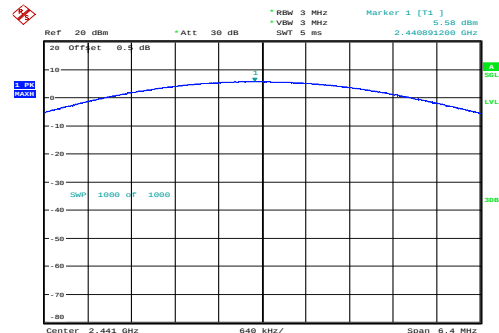
\pi/4 -DQPSK_Middle 5.58dBm
