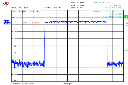
\pi/4 -DQPSK_Hopping_2DH3 1.687ms
