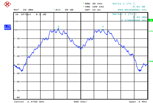
GFSK_High 0.998MHz
