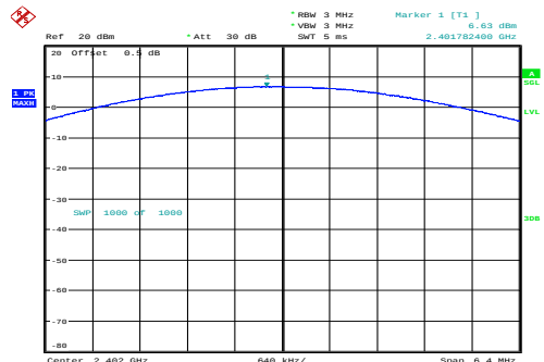
\pi/4 -DQPSK_Low 6.63dBm
