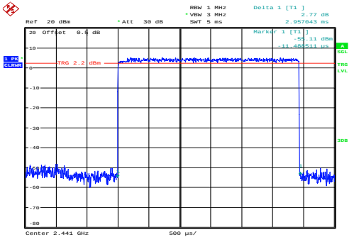
\pi/4 -DQPSK_Hopping_2DH5 2.957ms
