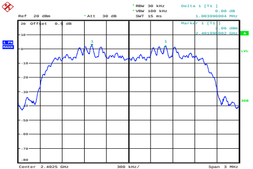
\pi/4 -DQPSK_Low 1.004MHz
