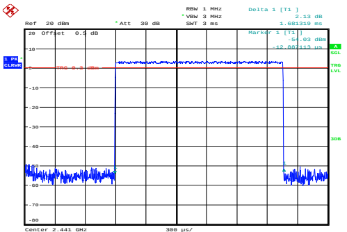
GFSK_Hopping_DH3 1.681ms
