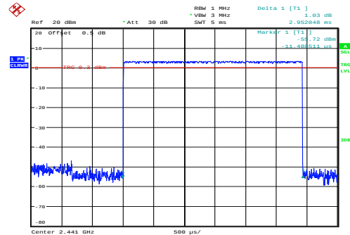
GFSK_Hopping_DH5 2.952ms
