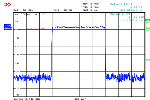
GFSK_Hopping_DH1 0.417ms
