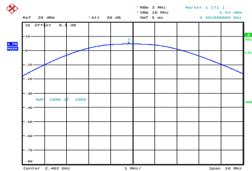
Low 4.54dBm
