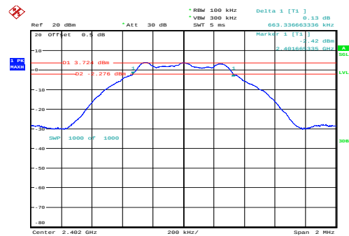
Low 0.663MHz
