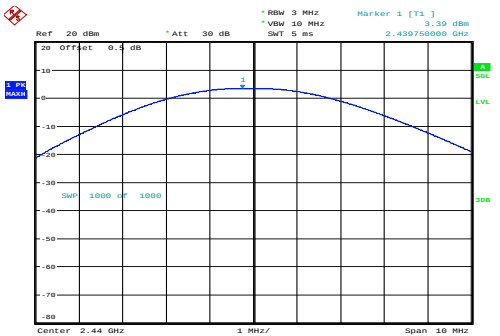
Middle 3.39dBm
