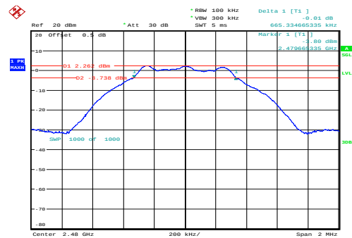
High 0.665MHz
