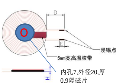
图三、线圈贴合磁片
