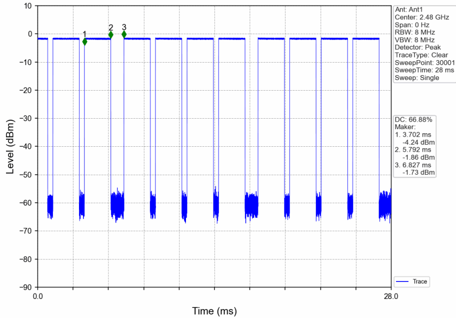
1M_HCH_2480MHz_DataRate=_Ant1_NTNV
