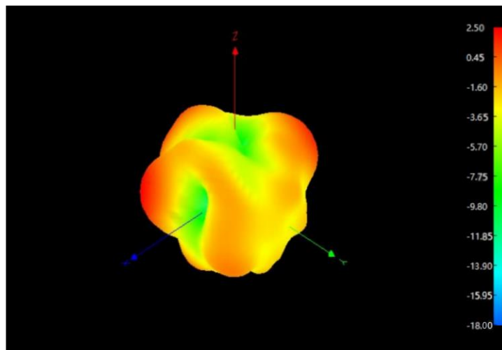
2480MHz 3D
