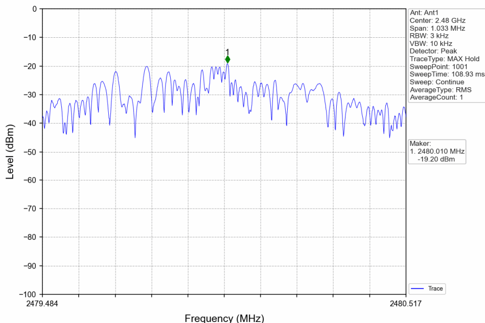
1M_HCH_2480MHz_DataRate=_Ant1_NTNV
