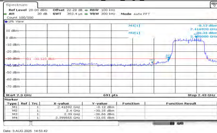
11AX20SISO_Ant1_Low_2412
