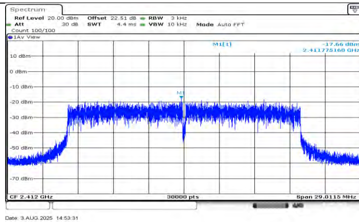
11AX20SISO_Ant1_2412
