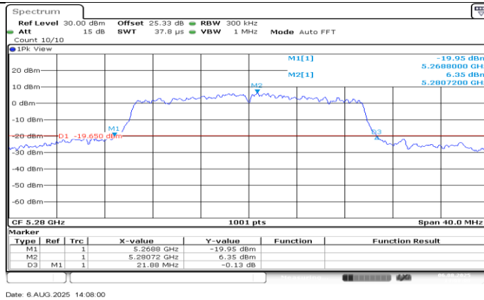
11AX20MIMO_Ant1_5280
