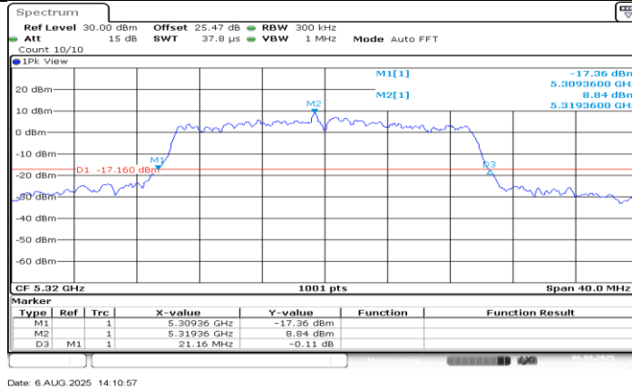
11AX20MIMO_Ant1_5320
