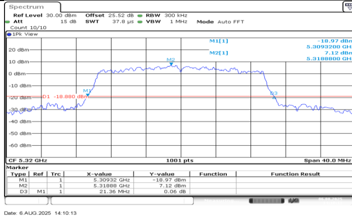
11AX20MIMO_Ant0_5320
