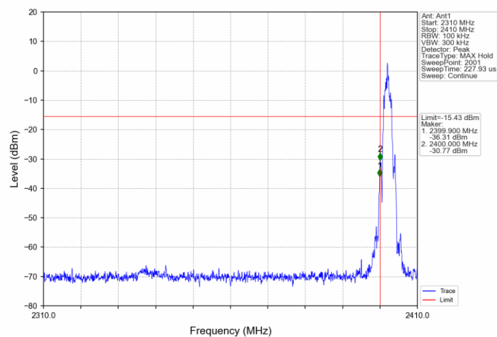
2M_LCH_2402MHz_ANT_B_NTNV
