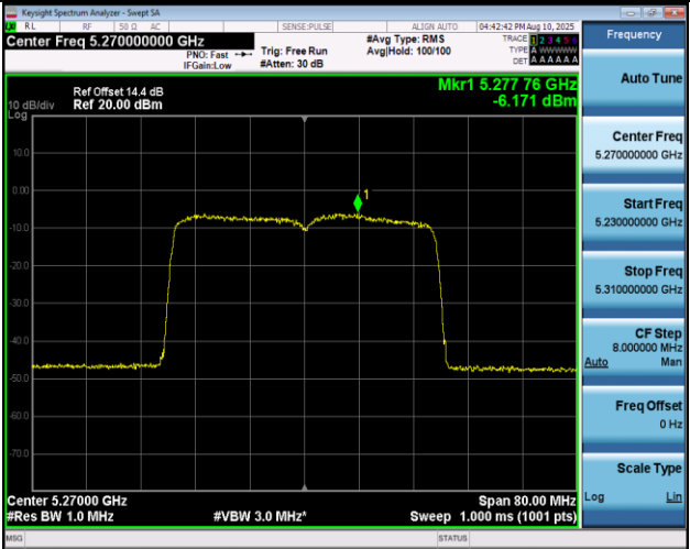
11AX40MIMO-Ant1-5270-PASS
