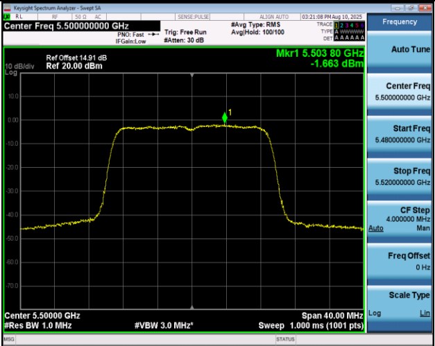
11AX20MIMO-Ant1-5500-PASS
