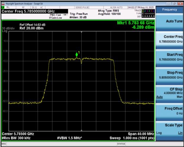
11AX20MIMO-Ant1-5785-PASS
