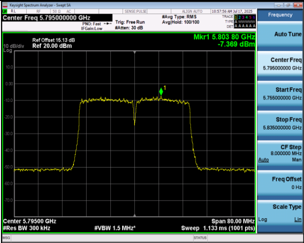
11N40MIMO-Ant1-5795-PASS
