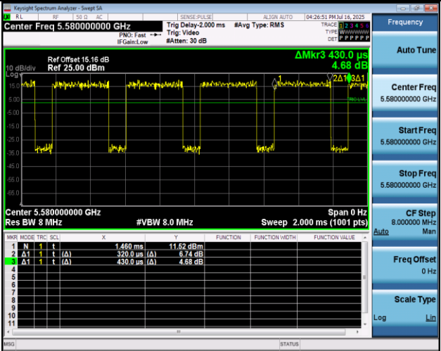
NTNV-11N20MIMO-Ant1-5580
