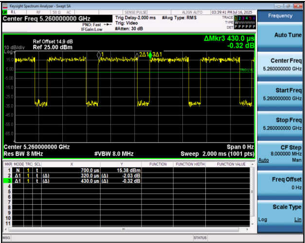
NTVN-11N20MIMO-Ant1-5260
