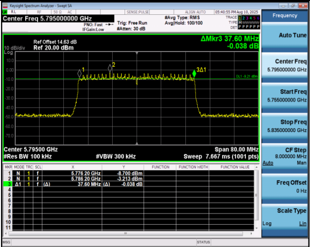
11AX40MIMO-Ant1-5795-PASS
