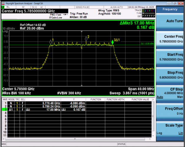
11AX20MIMO-Ant1-5785-PASS
