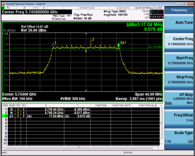
11AX20MIMO-Ant1-5745-PASS
