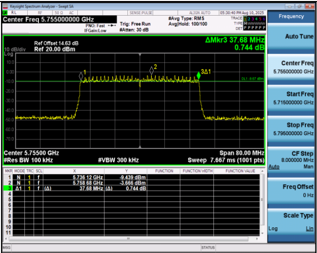
11AX40MIMO-Ant1-5755-PASS
