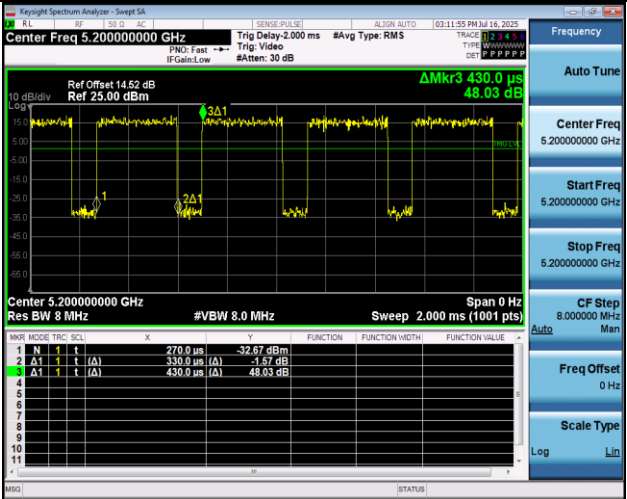
NTNV-11N20MIMO-Ant1-5200
