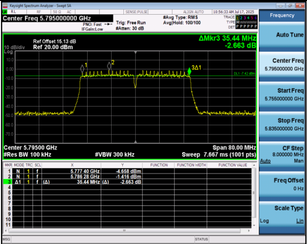
11N40MIMO-Ant1-5795-PASS
