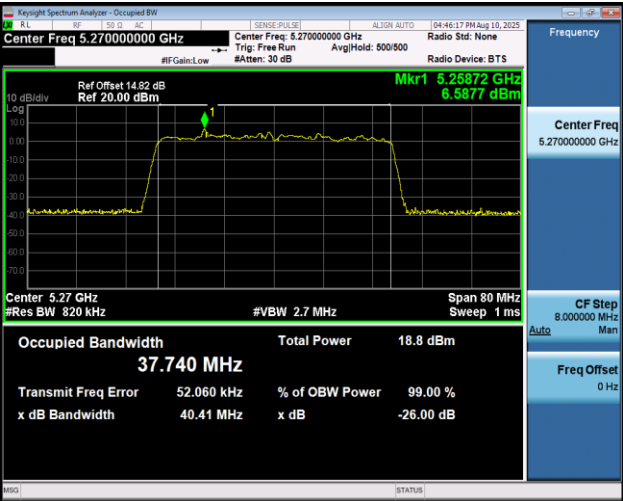
11AX40MIMO-Ant2-5270
