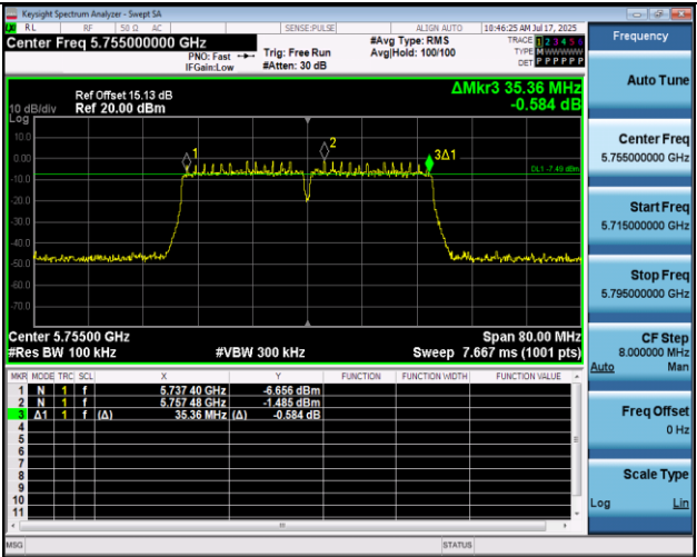
11N40MIMO-Ant1-5755-PASS
