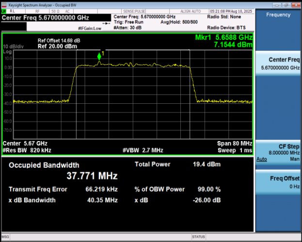
11AX40MIMO-Ant1-5670
