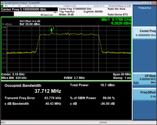
11AX40MIMO-Ant2-5190
