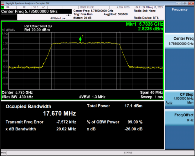
11AX20MIMO-Ant1-5785
