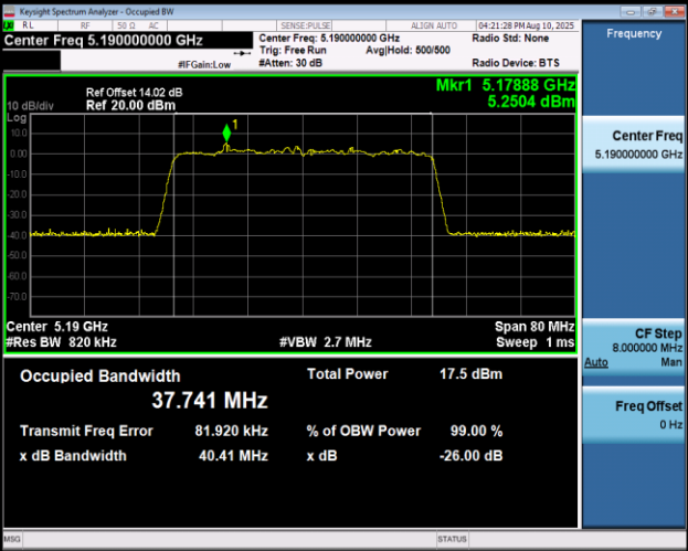
11AX40MIMO-Ant1-5190
