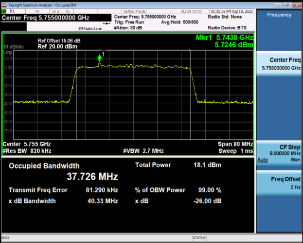
11AX40MIMO-Ant2-5755
