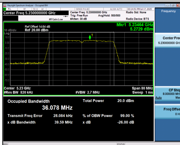
11AC40MIMO-Ant1-5230
