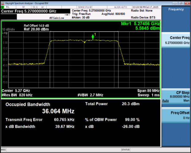
11AC40MIMO-Ant1-5270
