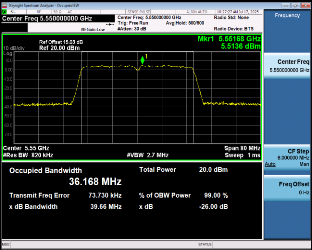
11N40MIMO-Ant1-5550
