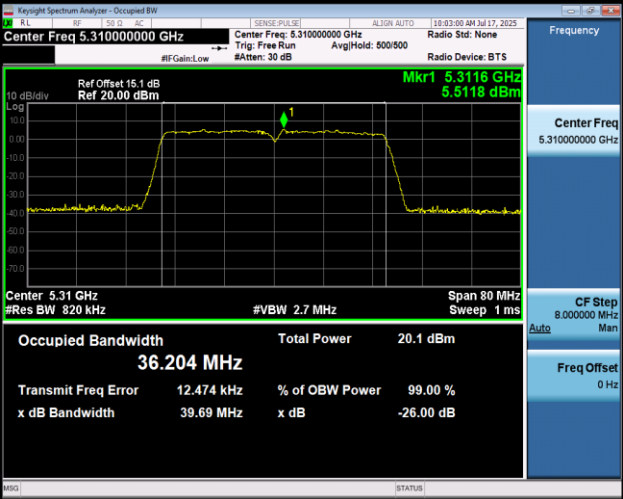
11N40MIMO-Ant1-5310
