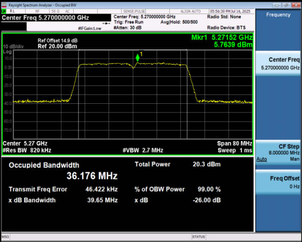
11N40MIMO-Ant1-5270
