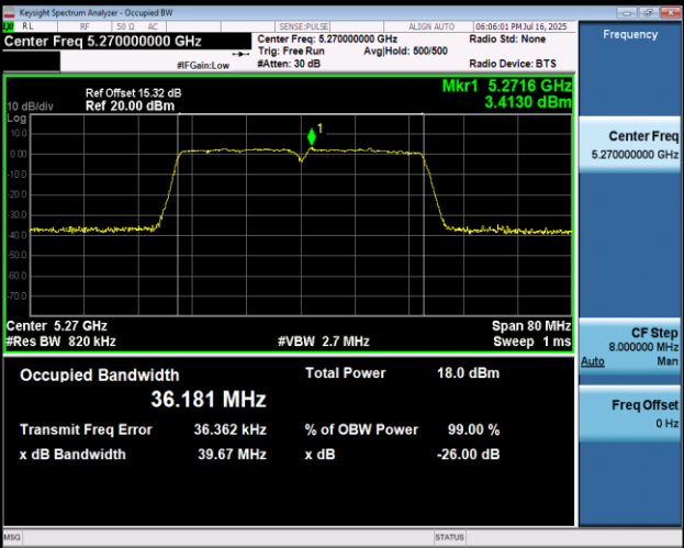
11N40MIMO-Ant2-5270
