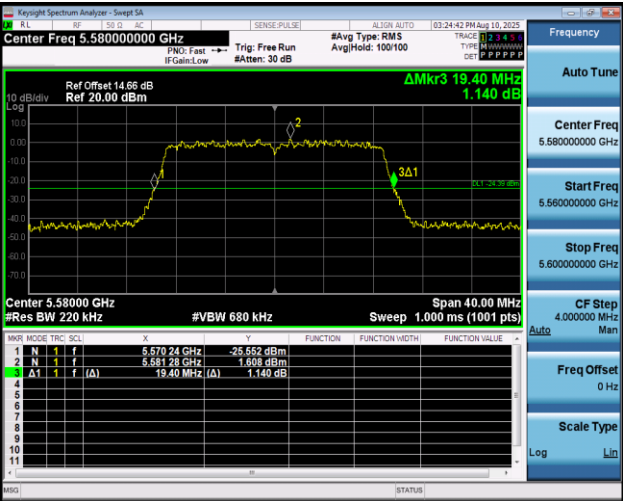
11AX20MIMO-Ant1-5580
