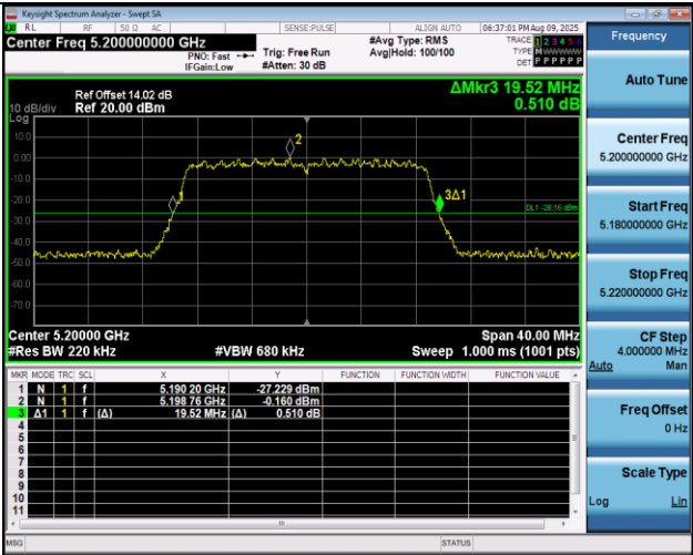
11AX20MIMO-Ant1-5200
