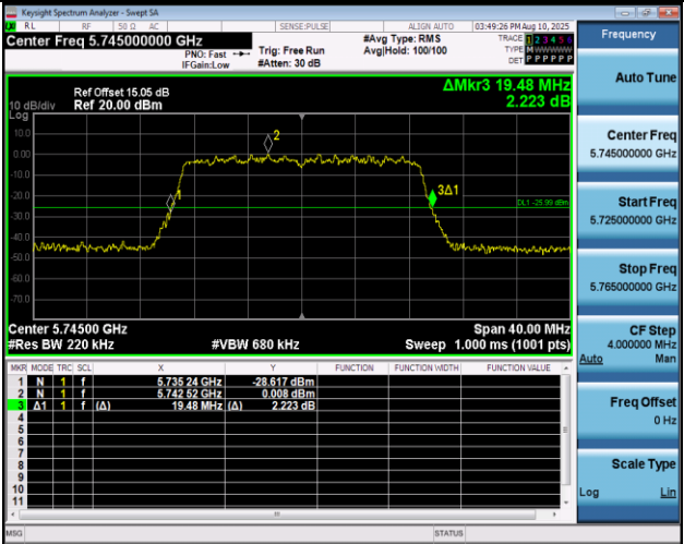
11AX20MIMO-Ant2-5745
