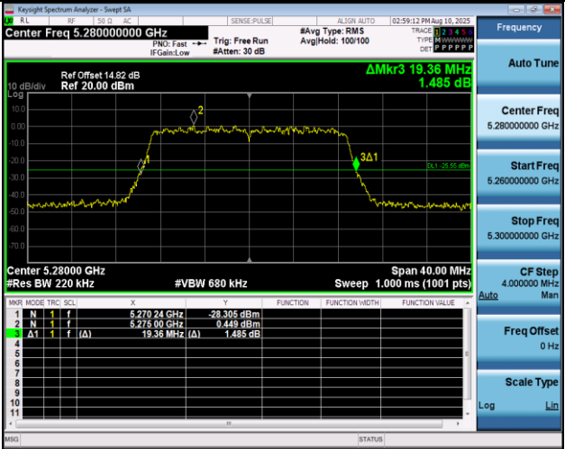
11AX20MIMO-Ant2-5280
