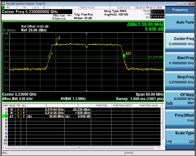
11AC40MIMO-Ant1-5230
