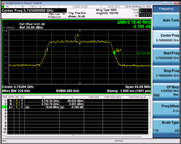
11AX20MIMO-Ant1-5745
