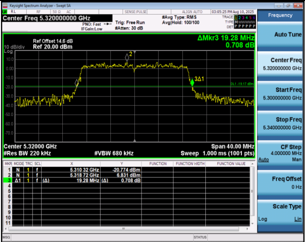
11AX20MIMO-Ant1-5320
