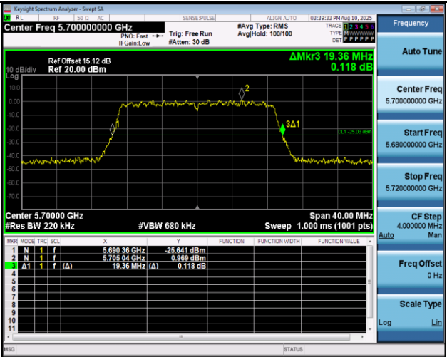
11AX20MIMO-Ant2-5700
