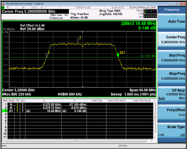
11AX20MIMO-Ant1-5280
