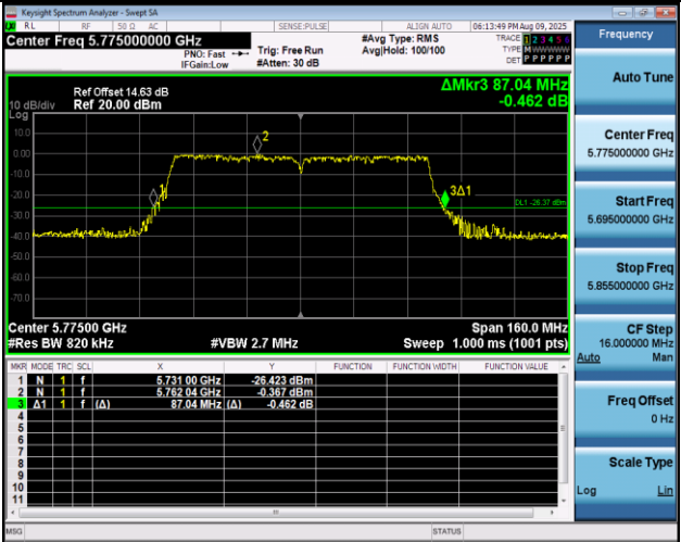
11AC80MIMO-Ant1-5775
