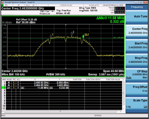
11B-Ant2-2462-PASS
