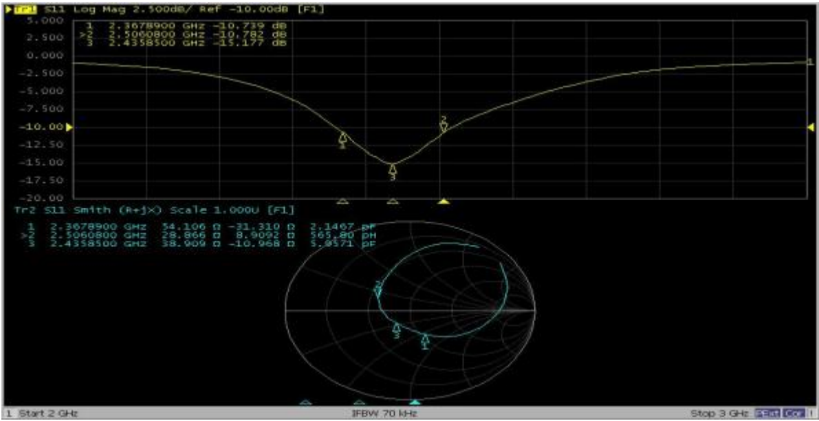
图NormalModule天线 s11
