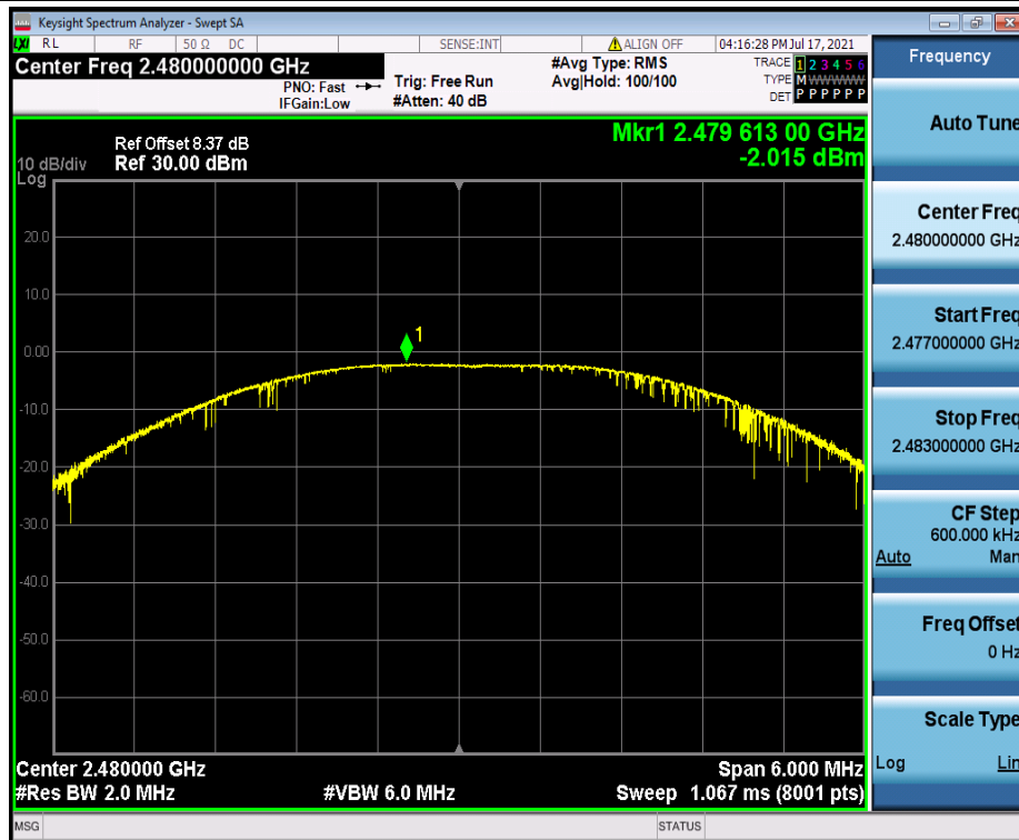
BLE_2M_Ant1_2480
