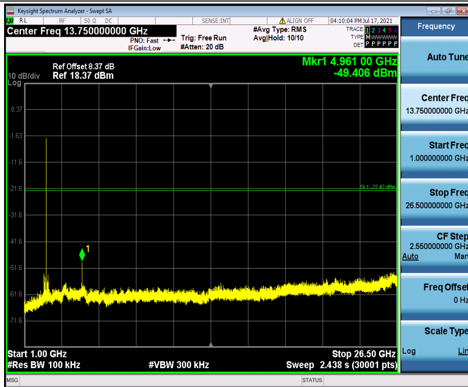
BLE_1M_Ant1_2480_1000~26500
