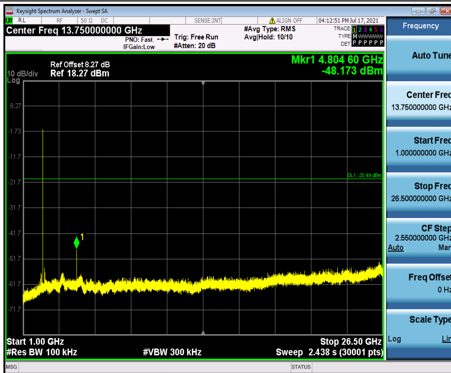
BLE_2M_Ant1_2402_1000~26500
