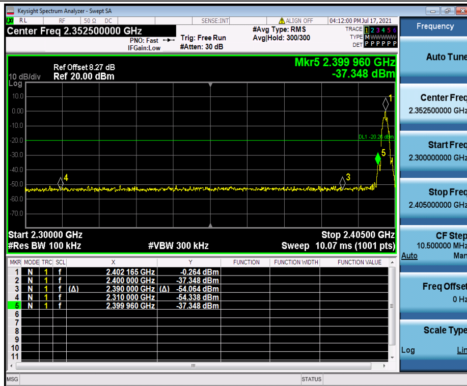
BLE_2M_Ant1_Low_2402
