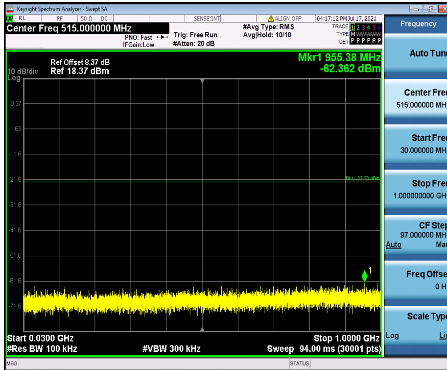
BLE_2M_Ant1_2480_30~1000
