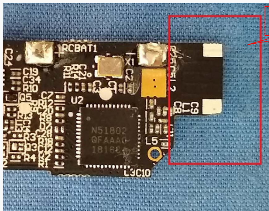
BLE Antenna
