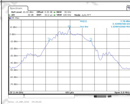
99% Bandwidth Mode2 CH 06
