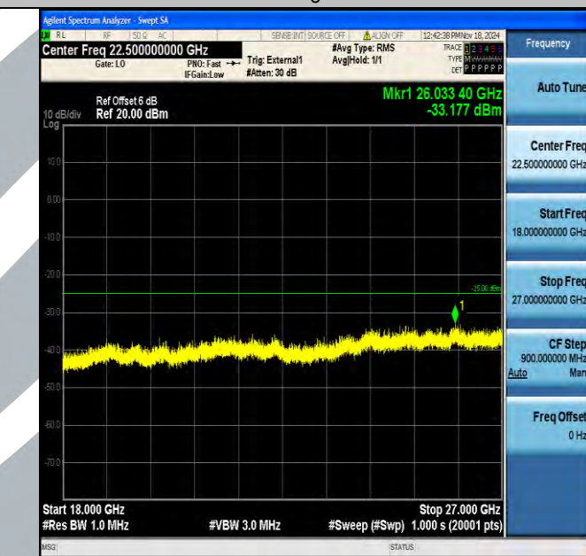
Band41_20MHz_16QAM_40140_1RB#0_18000~27000_18000~27000
