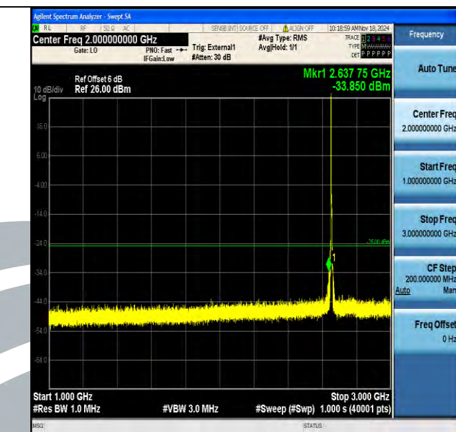
Band41 5MHz 16QAM 41215 1RB#0 1000~3000 1000~3000
