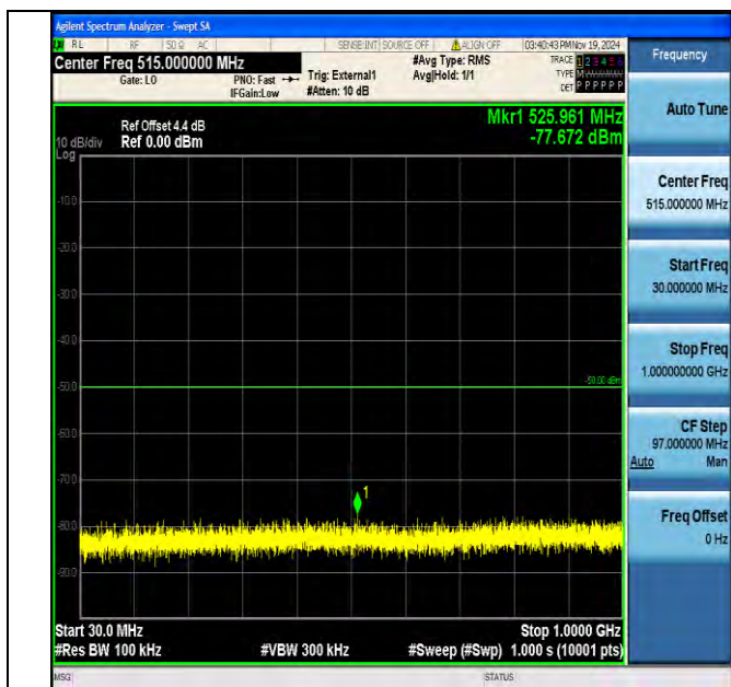
Band40 5MHz QPSK 38725 1RB#0 30~1000 30~1000
