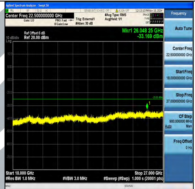
Band41_15MHz_16QAM_40590_1RB#0_18000~27000_18000~27000
