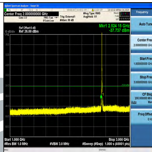
Band41 5MHz QPSK 40065 1RB#0 1000~3000 1000~3000
