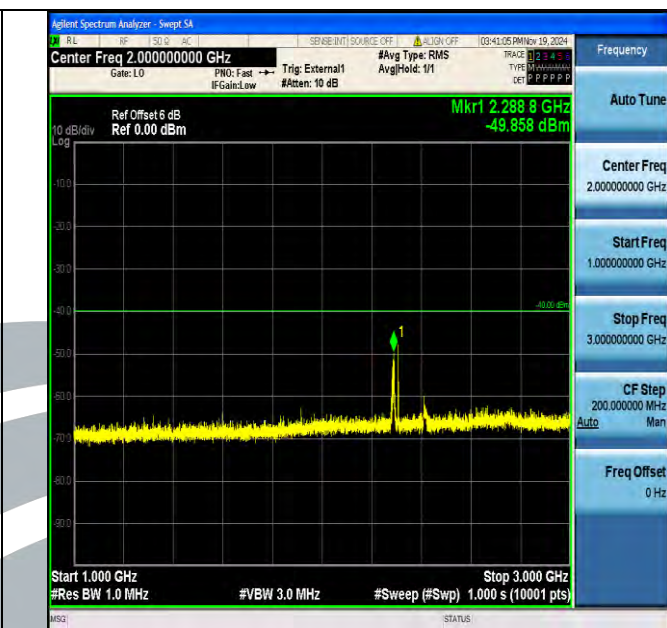
Band40 5MHz QPSK 38725 1RB#0 1000~3000 1000~3000
