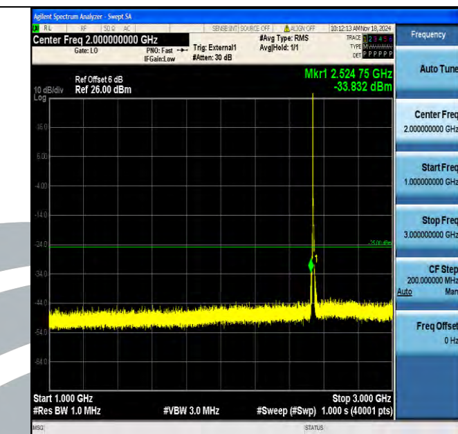
Band41 5MHz 16QAM 40065 1RB#0 1000~3000 1000~3000
