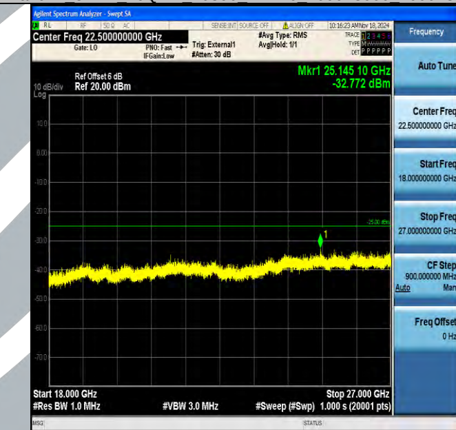
Band41_5MHz_16QAM_40590_1RB#0_18000~27000_18000~27000
