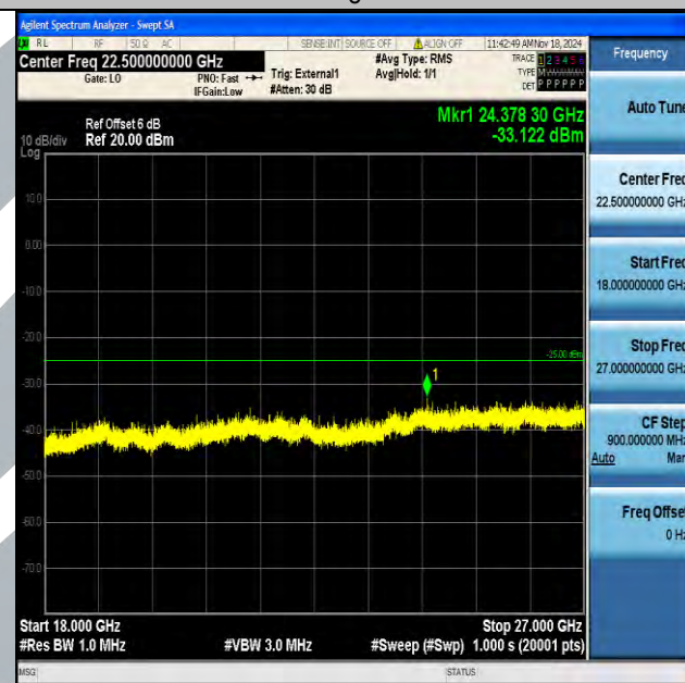
Band41_10MHz_16QAM_41190_1RB#0_18000~27000_18000~27000
