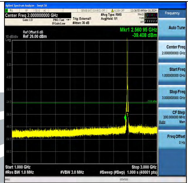
Band41 10MHz QPSK 40590 1RB#0 1000~3000 1000~3000
