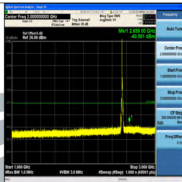
Band41 10MHz QPSK 40090 1RB#0 1000~3000 1000~3000
