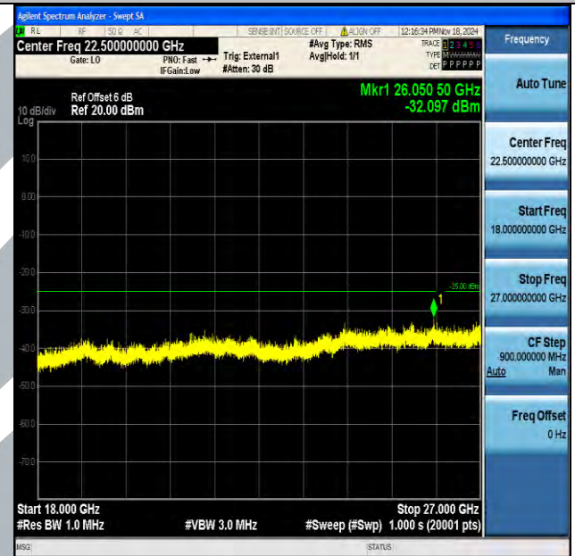
Band41_15MHz_16QAM_41165_1RB#0_18000~27000_18000~27000
