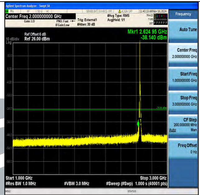
Band41 10MHz QPSK 41190 1RB#0 1000~3000 1000~3000
