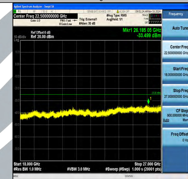
Band38_15MHz_16QAM_38175_1RB#0_18000~27000_18000~27000
