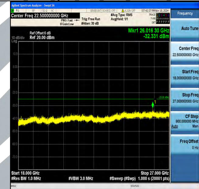
Band7_20MHz_QPSK_20850_1RB#0_18000~27000_18000~27000
