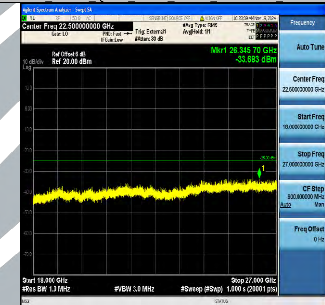
Band38_20MHz_QPSK_38150_1RB#0_18000~27000_18000~27000
