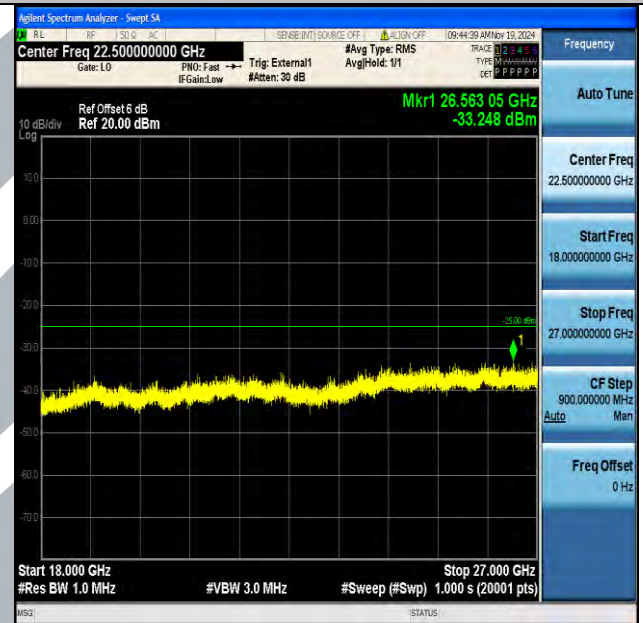
Band38_15MHz_16QAM_37825_1RB#0_18000~27000_18000~27000
