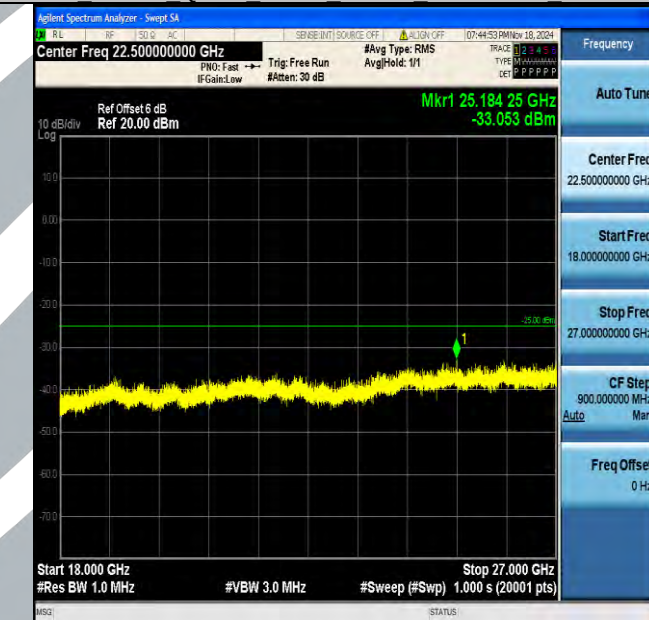
Band7_20MHz_QPSK_21350_1RB#0_18000~27000_18000~27000
