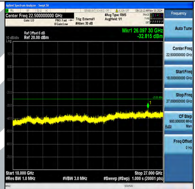
Band38_10MHz_16QAM_38000_1RB#0_18000~27000_18000~27000
