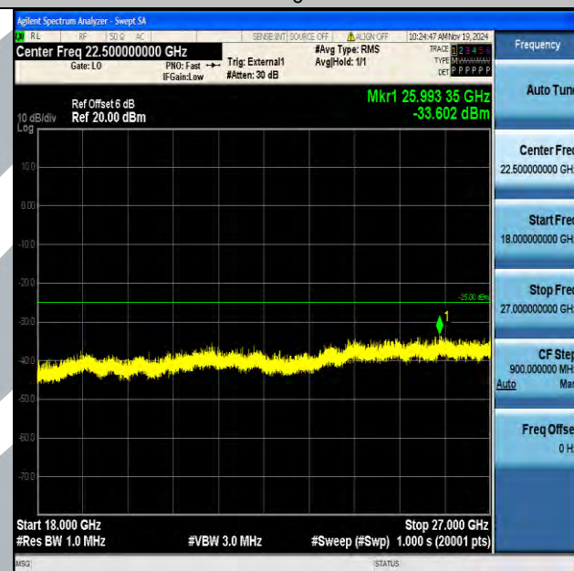
Band38_20MHz_16QAM_38150_1RB#0_18000~27000_18000~27000
