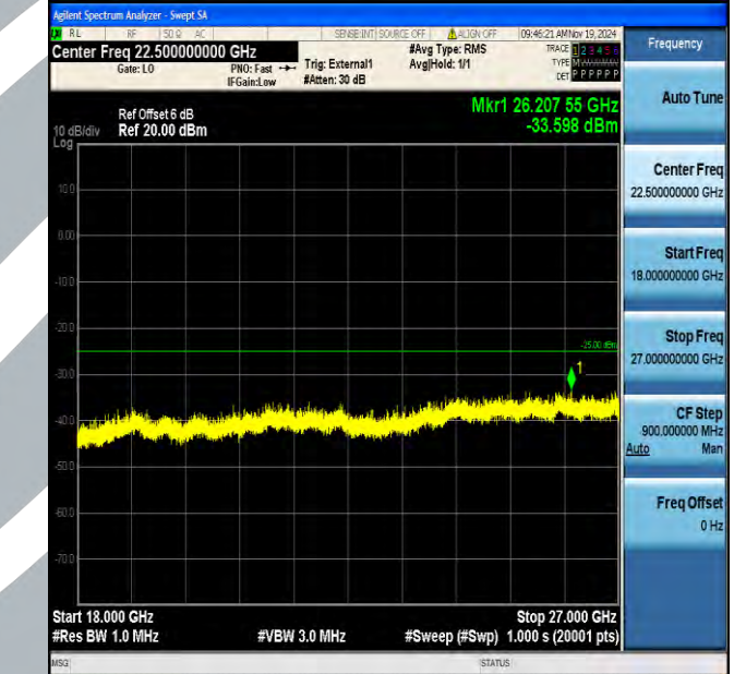
Band38_15MHz_QPSK_38000_1RB#0_18000~27000_18000~27000
