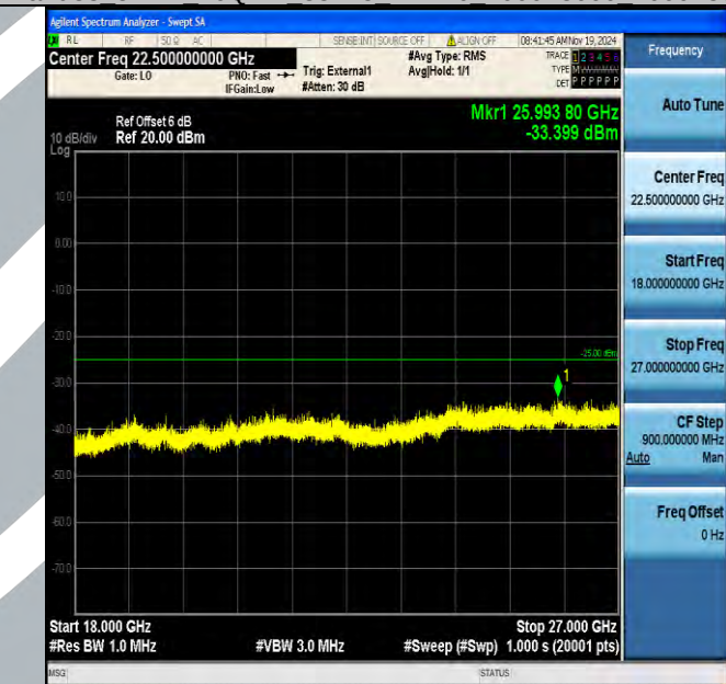
Band38_5MHz_16QAM_38225_1RB#0_18000~27000_18000~27000
