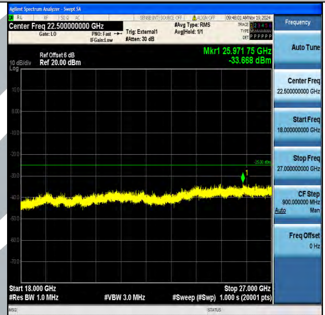
Band38_15MHz_16QAM_38000_1RB#0_18000~27000_18000~27000
