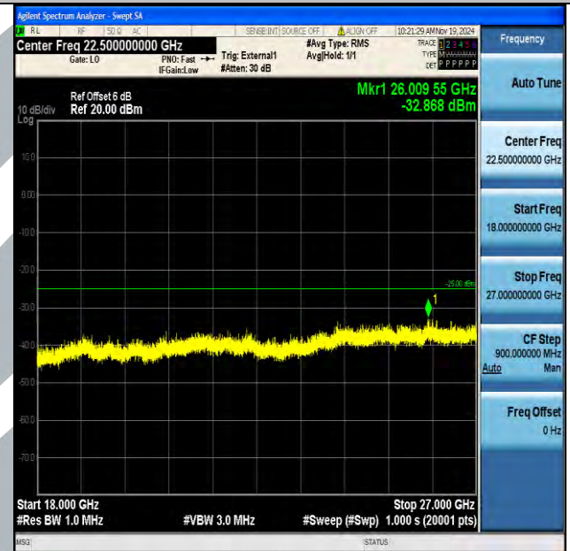
Band38_20MHz_16QAM_38000_1RB#0_18000~27000_18000~27000
