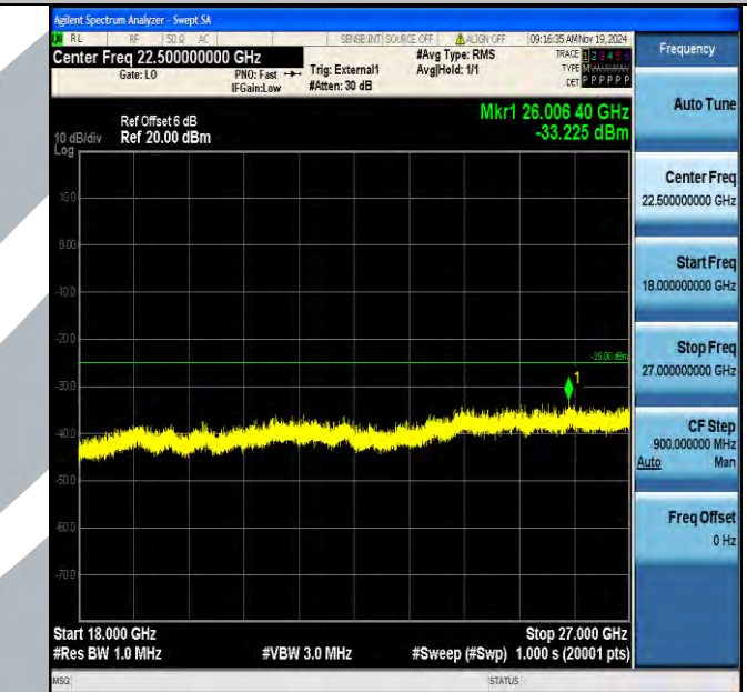
Band38_10MHz_16QAM_38200_1RB#0_18000~27000_18000~27000
