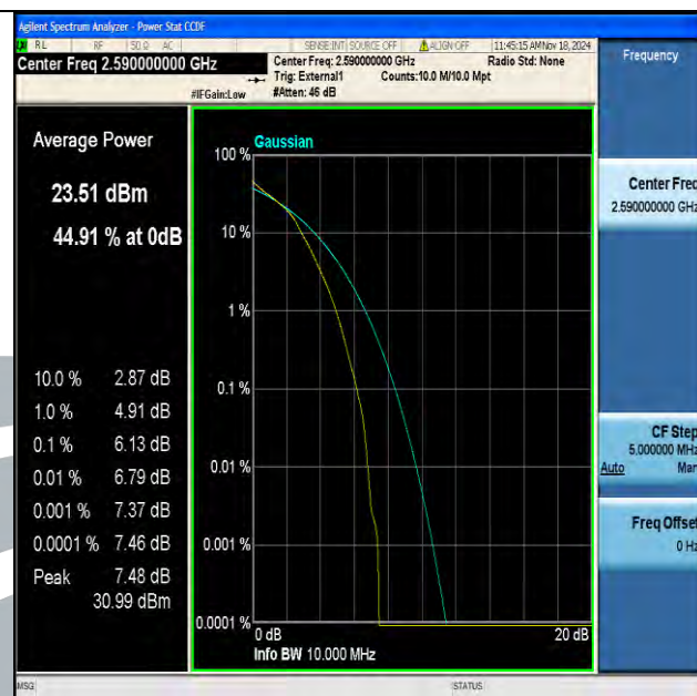
Band41(2535-2655)-10MHz-16QAM-40590-50RB#0-PASS
