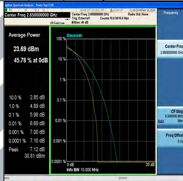
Band41(2535-2655)-10MHz-16QAM-41190-50RB#0-PASS
