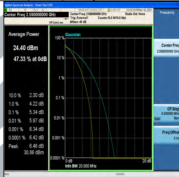
Band41(2535-2655)-20MHz-QPSK-40590-100RB#0-PASS
