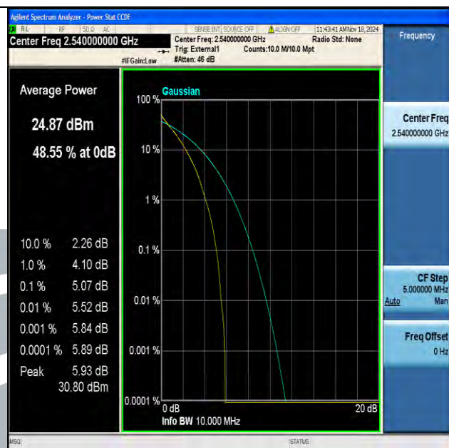
Band41(2535-2655)-10MHz-QPSK-40090-50RB#0-PASS
