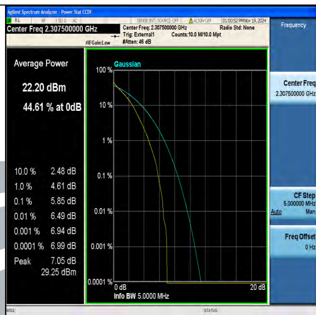
Band40(2305-2315)-5MHz-QPSK-38725-25RB#0-PASS
