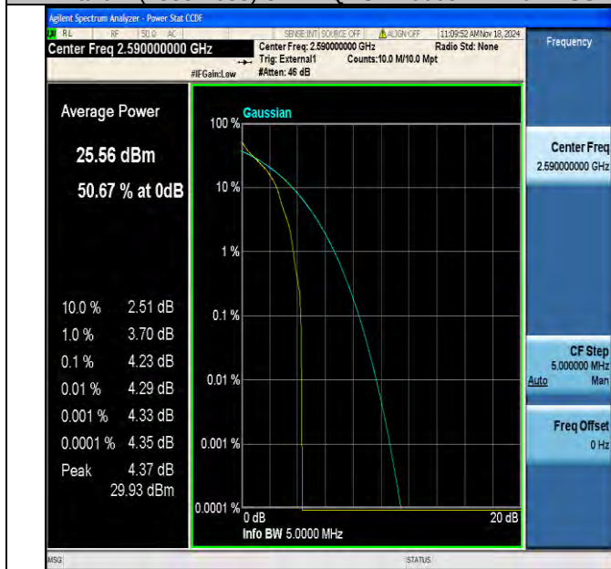
Band41(2535-2655)-5MHz-QPSK-40590-1RB#0-PASS
