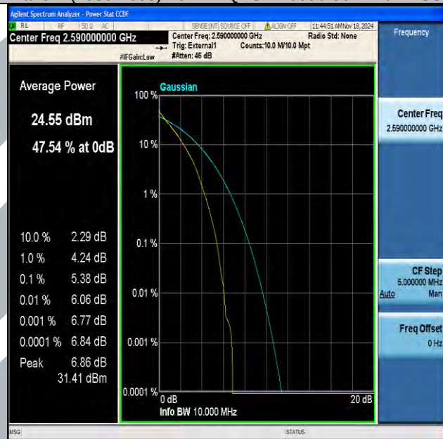
Band41(2535-2655)-10MHz-QPSK-40590-50RB#0-PASS
