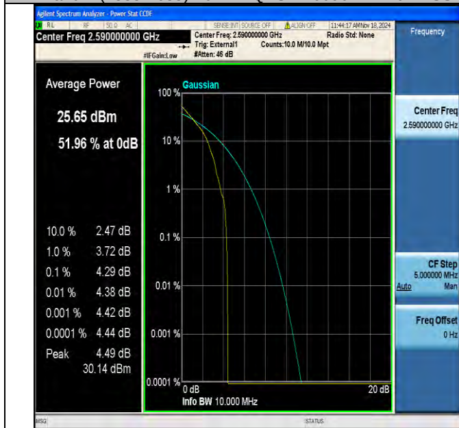
Band41(2535-2655)-10MHz-QPSK-40590-1RB#0-PASS
