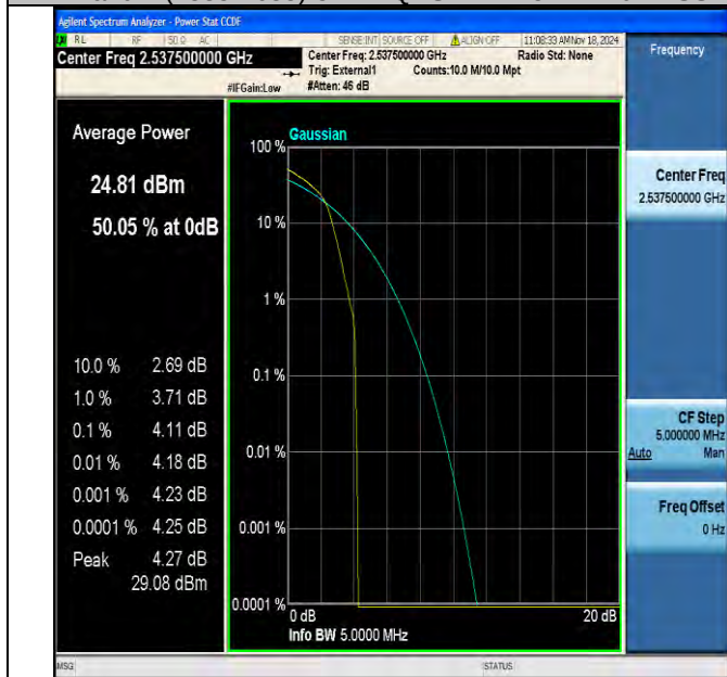
Band41(2535-2655)-5MHz-16QAM-40065-1RB#0-PASS
