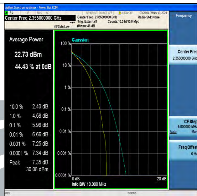
Band40(2350-2360)-10MHz-QPSK-39200-50RB#0-PASS
