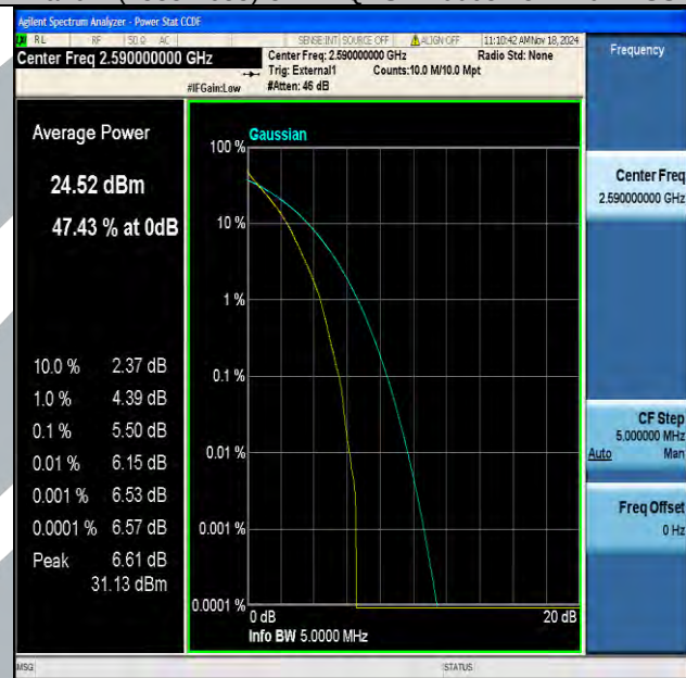
Band41(2535-2655)-5MHz-QPSK-40590-25RB#0-PASS
