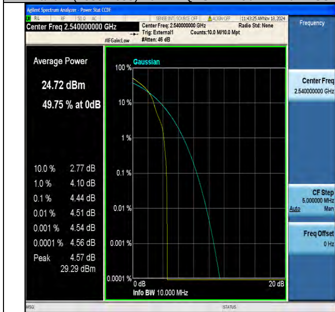
Band41(2535-2655)-10MHz-16QAM-40090-1RB#0-PASS
