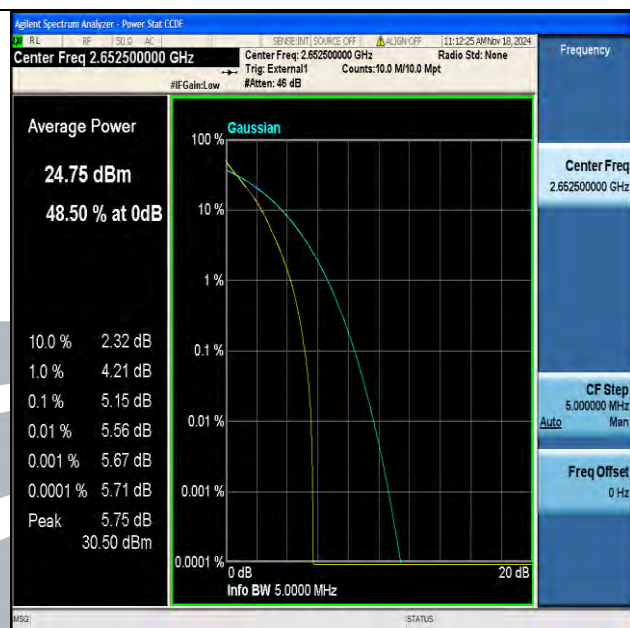
Band41(2535-2655)-5MHz-QPSK-41215-25RB#0-PASS
