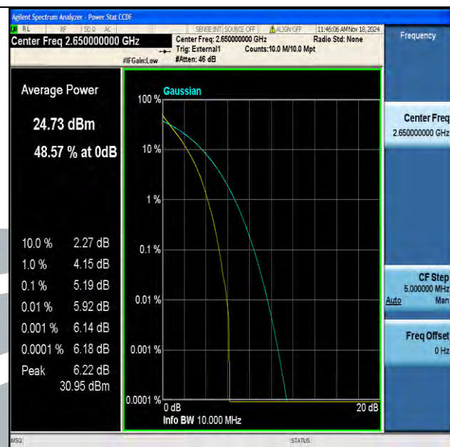
Band41(2535-2655)-10MHz-QPSK-41190-50RB#0-PASS
