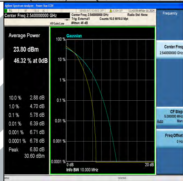
Band41(2535-2655)-10MHz-16QAM-40090-50RB#0-PASS
