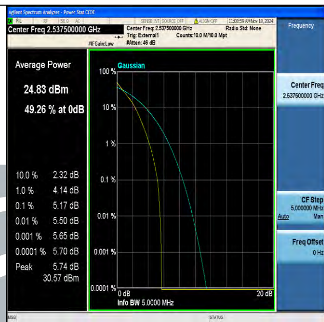
Band41(2535-2655)-5MHz-QPSK-40065-25RB#0-PASS
