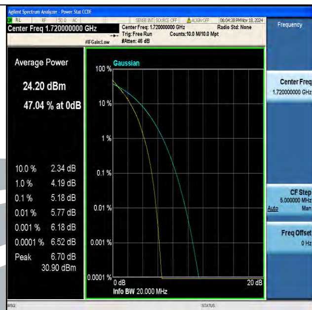
Band4-20MHz-QPSK-20050-100RB#0-PASS
