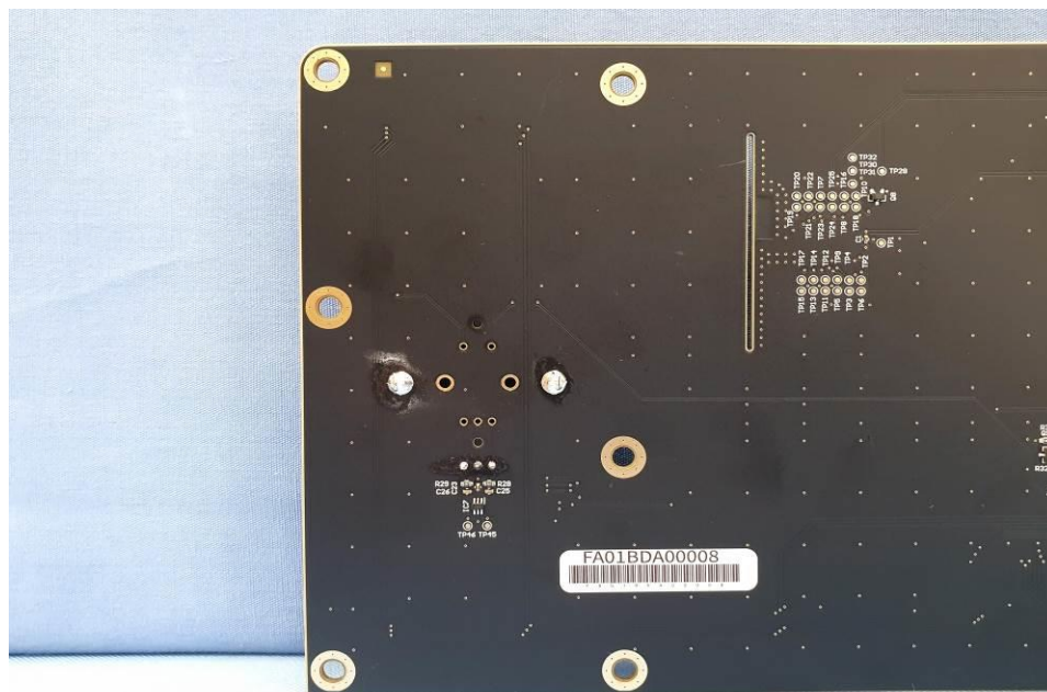
EUT Photo (4)
