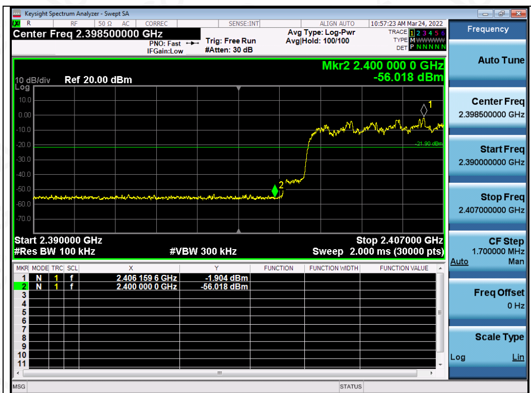
Test_Graph_EDR_HOP_ANT1_NA_3Mbps_Lower Band Edge Emission
