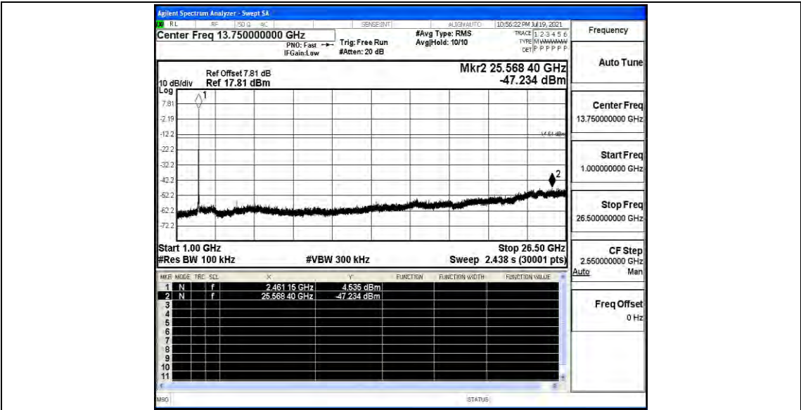
11B_Ant1_2462_1000~26500
