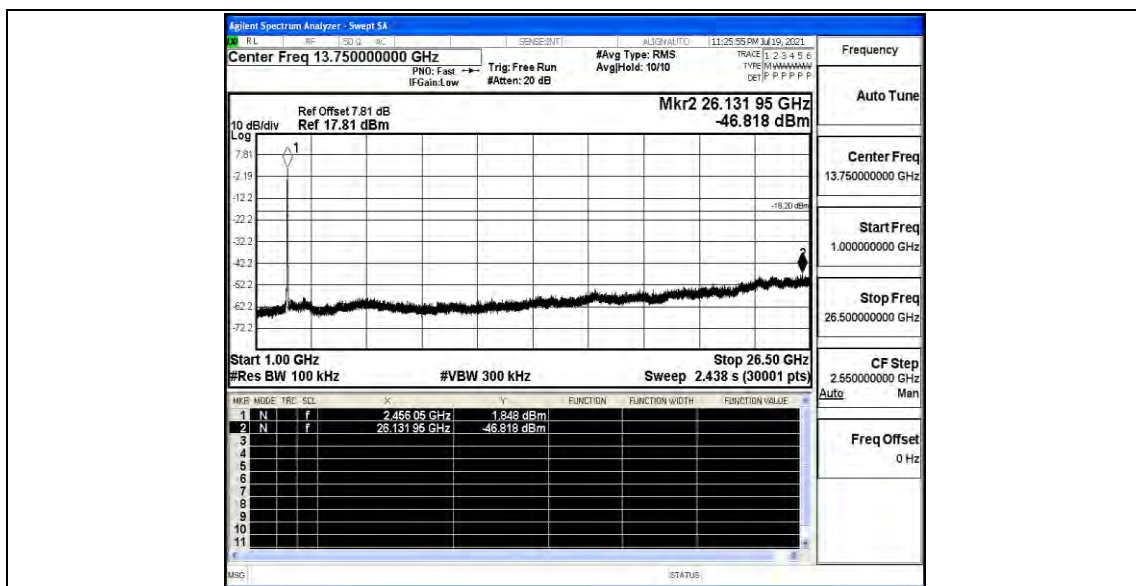
11N20ISO_Ant1_2462_1000~26500
