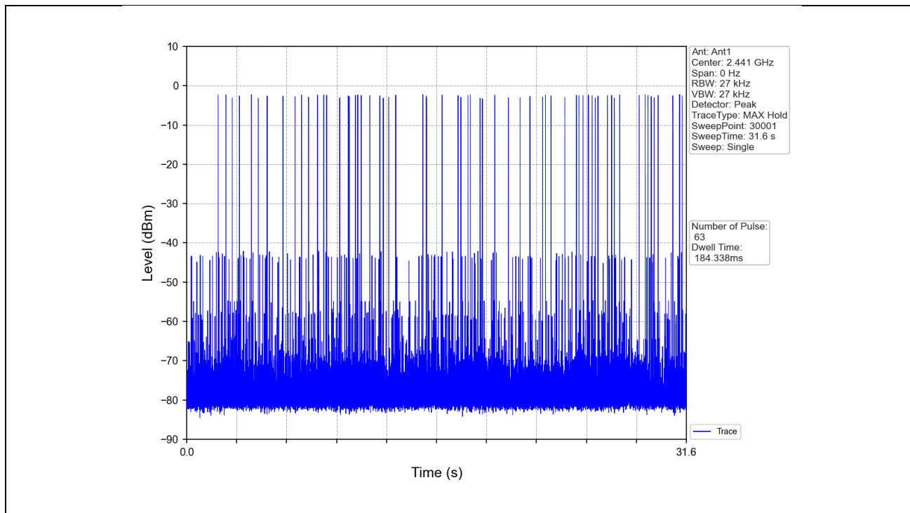
8DPSK_3DH1_HOPP_Ant1_NTNV
