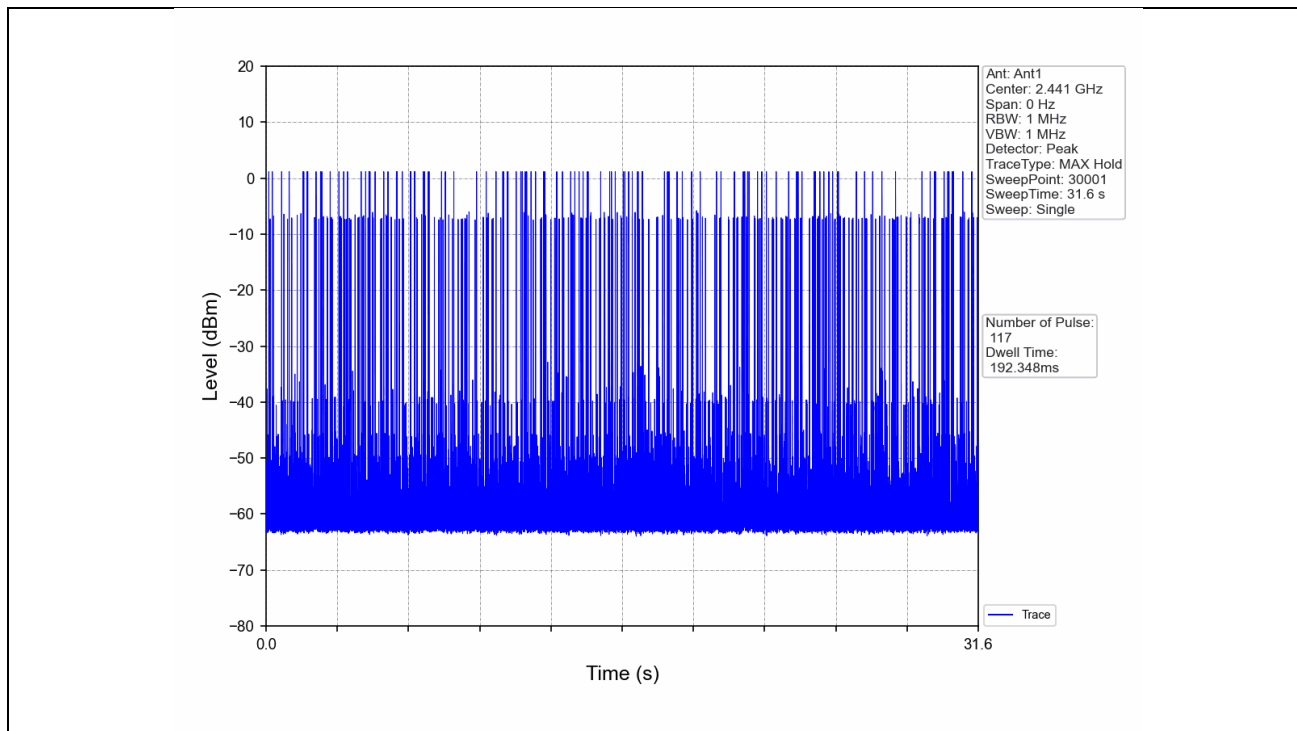
GFSK_DH5_HOPP_Ant1_NTNV
