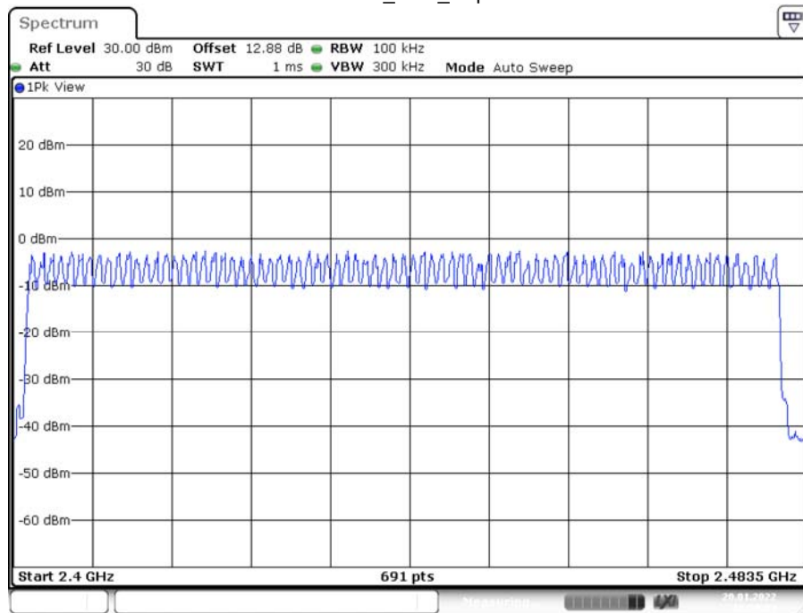
2DH1_Ant1_Hop
