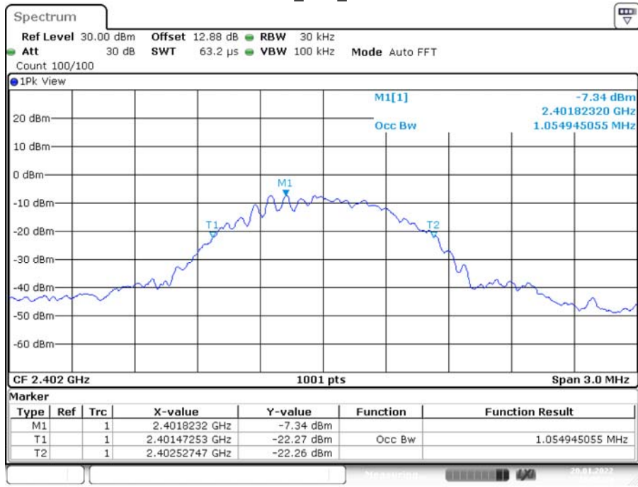
DH1_Ant1_2402
