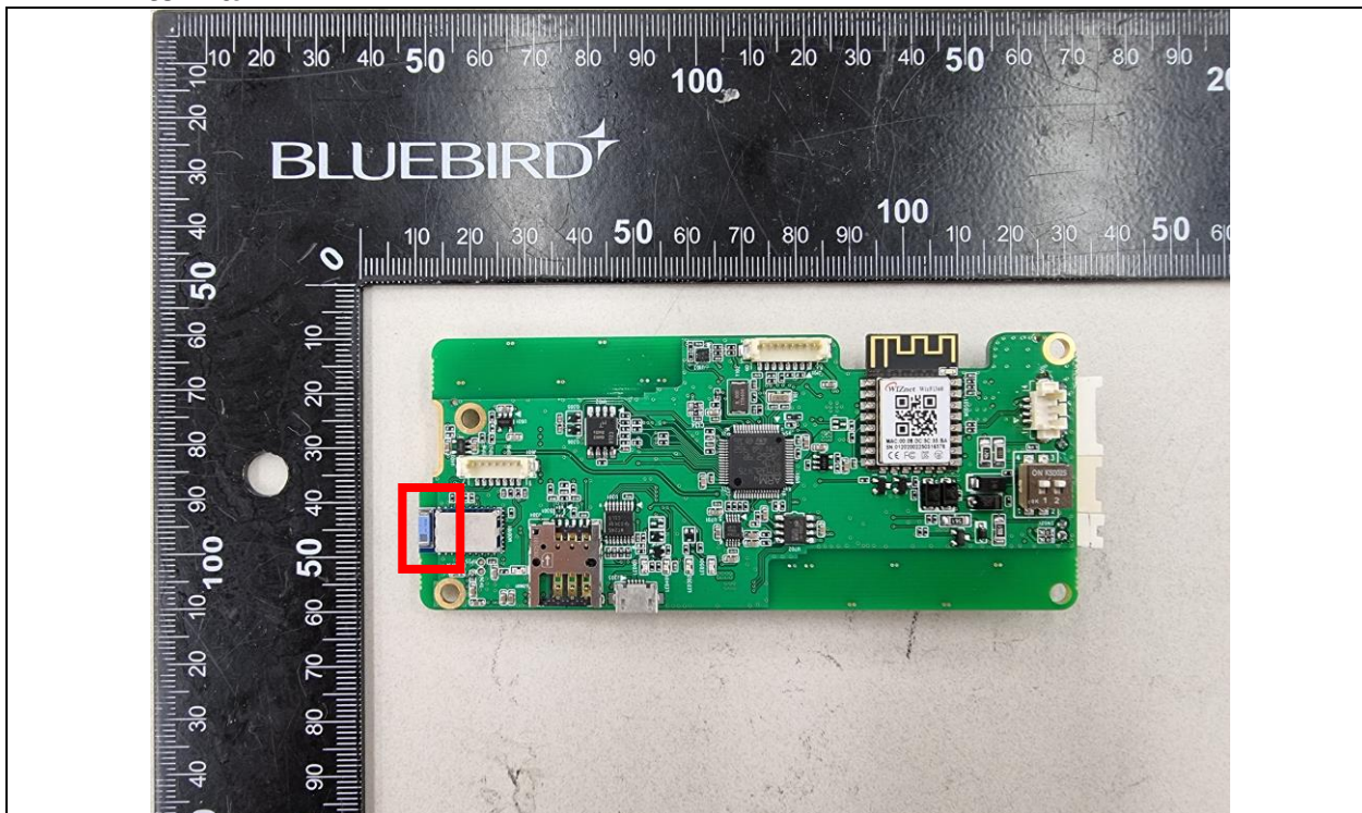
BLE Antenna
