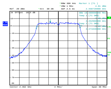
n20_2462MHz_Chain 0
