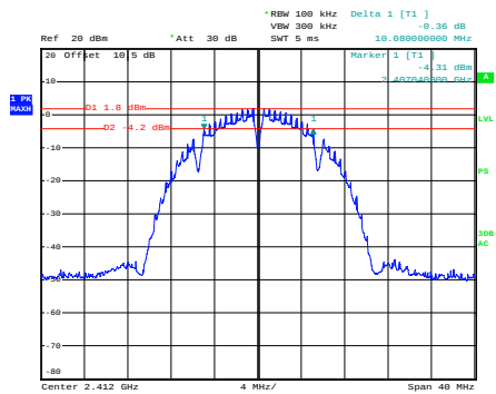
b_2412MHz_Chain 0
