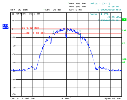
b_2462MHz_Chain 0
