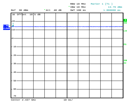
b_2437MHz_Chain 0
