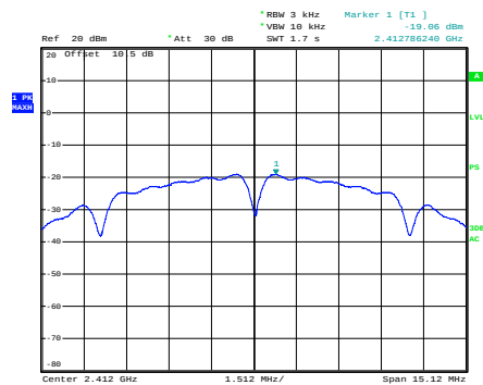
b_2412MHz_Chain 0
