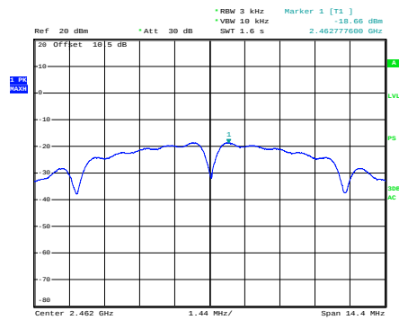
b_2462MHz_Chain 0
