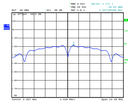
b_2437MHz_Chain 0
