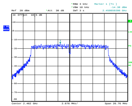
n20_2462MHz_Chain 0
