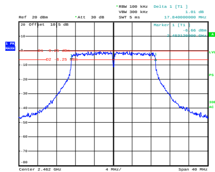
n20_2462MHz_Chain 0
