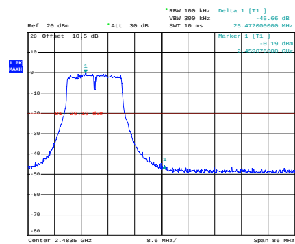
n20_2462MHz_Chain 0
