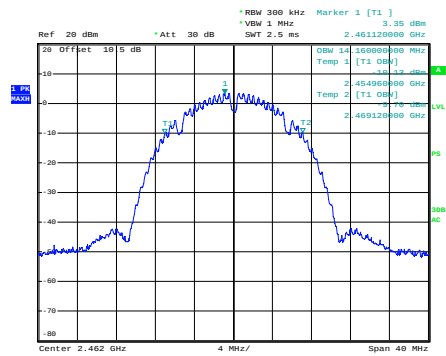
b_2462MHz_Chain 0
