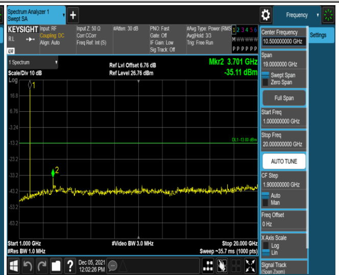
Band2-1.4MHz-QPSK-18900-1RB#0-Range2:1000~2 0000MHz
