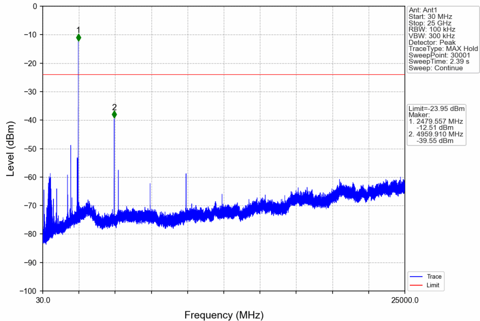
GFSK HCH 2480MHz Ant1 NTN
