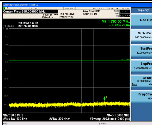
Band4-3MHz-QPSK-19965-1-0-Low-30-1000--60.6-PASS
