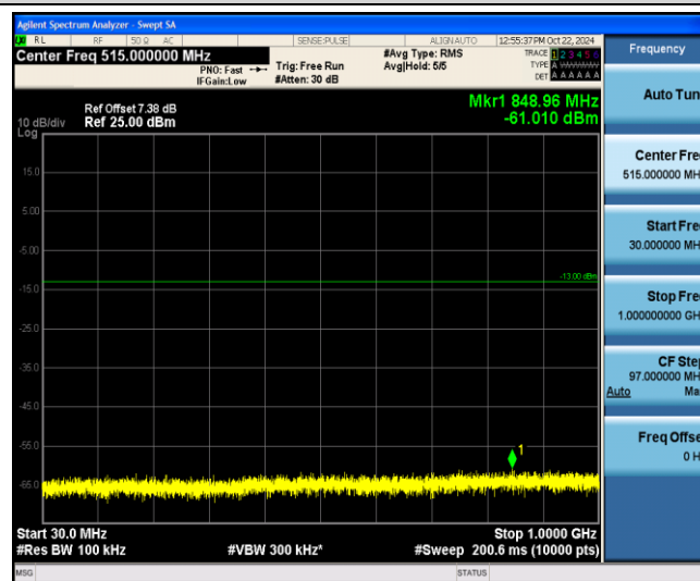
Band4-3MHz-QPSK-20175-1-0-Low-30-1000--61.01-PASS
