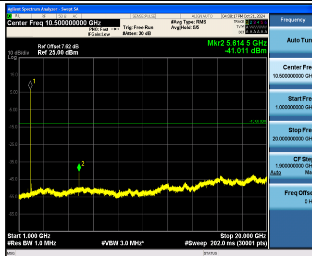
Band2-20MHz-16QAM-18900-1-0-Low-1000-20000--41.01-PASS
