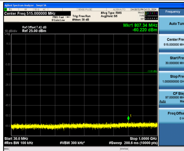
Band2-20MHz-QPSK-19100-1-0-Low-30-1000--60.22-PASS
