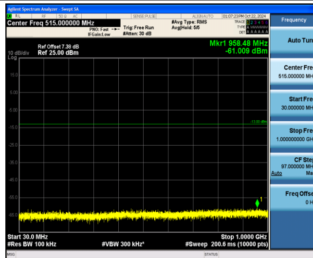
Band4-3MHz-16QAM-20385-1-0-Low-30-1000--61.01-PASS
