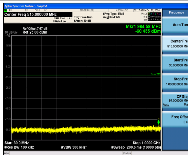
Band4-10MHz-QPSK-20000-1-0-Low-30-1000--60.44-PASS
