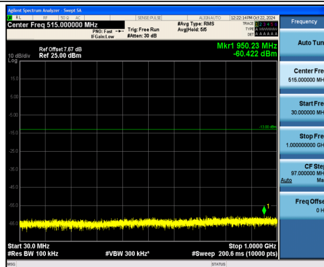
Band4-1.4MHz-QPSK-19957-1-0-Low-30-1000--60.42-PASS
