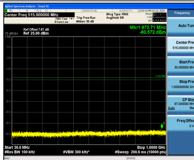
Band4-3MHz-16QAM-19965-1-0-Low-30-1000--60.57-PASS
