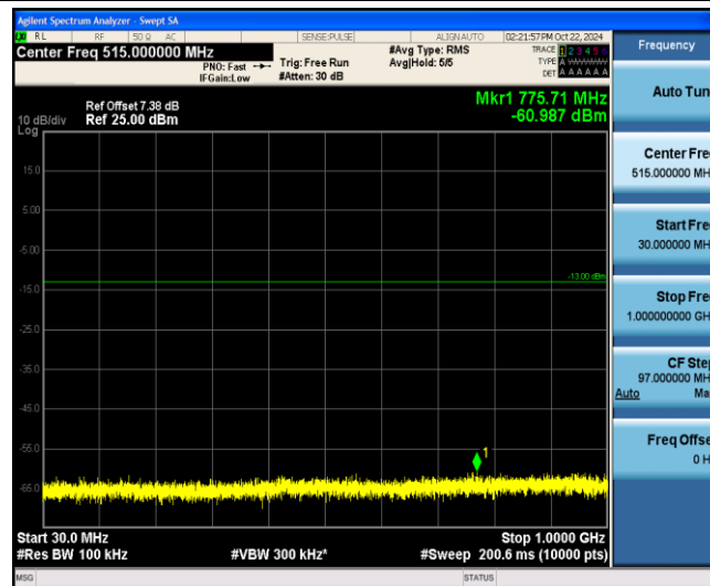
Band4-10MHz-QPSK-20350-1-0-Low-30-1000--60.99-PASS
