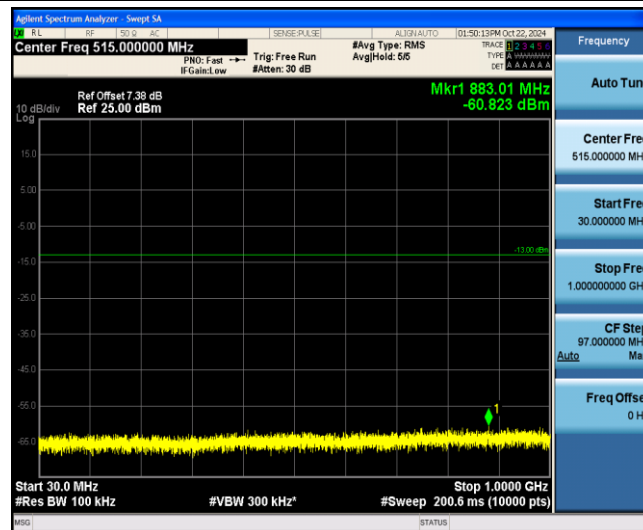
Band4-5MHz-QPSK-20375-1-0-Low-30-1000--60.82-PASS
