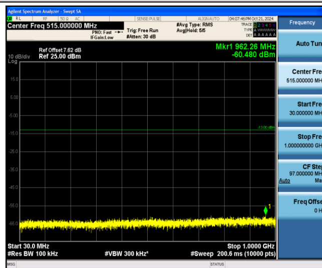
Band2-20MHz-QPSK-18900-1-0-Low-30-1000--60.48-PASS
