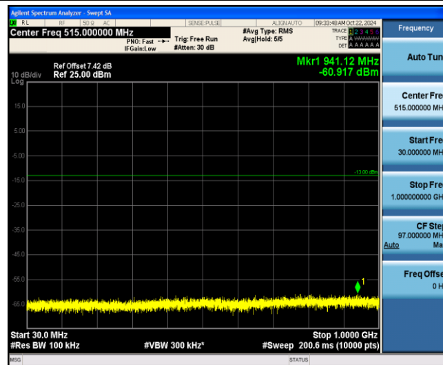
Band2-3MHz-QPSK-19185-1-0-Low-30-1000--60.92-PASS
