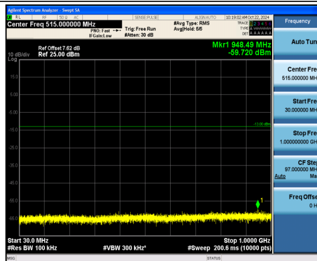
Band2-5MHz-QPSK-18625-1-0-Low-30-1000--59.72-PASS
