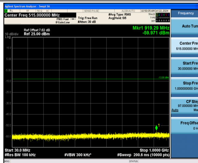
Band2-10MHz-QPSK-18650-1-0-Low-30-1000--59.97-PASS
