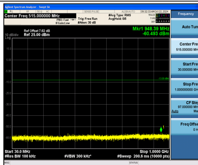
Band2-3MHz-QPSK-18900-1-0-Low-30-1000--60.49-PASS
