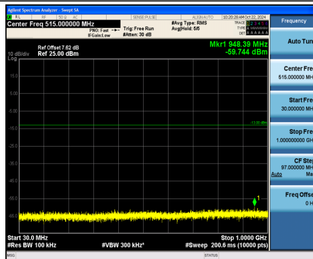
Band2-5MHz-16QAM-18900-1-0-Low-30-1000--59.74-PASS
