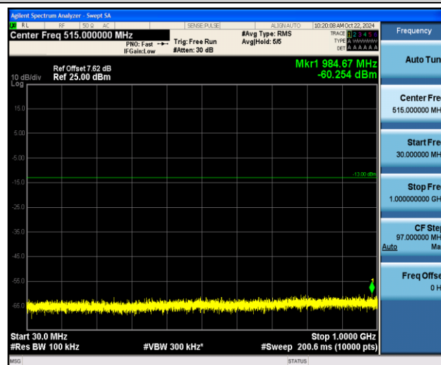
Band2-5MHz-QPSK-18900-1-0-Low-30-1000--60.25-PASS
