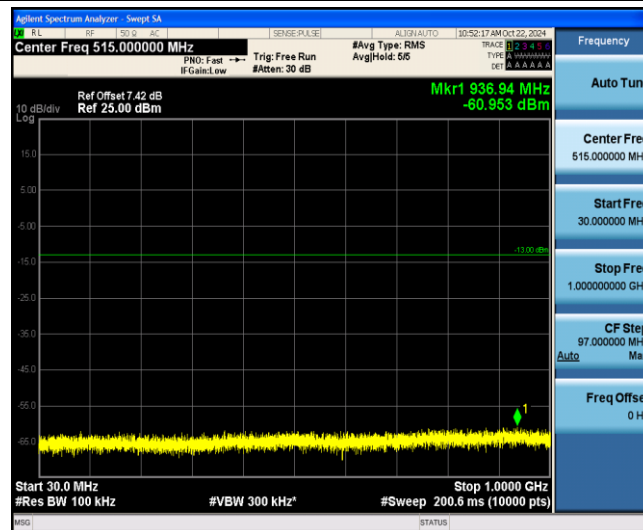
Band2-10MHz-QPSK-19150-1-0-Low-30-1000--60.95-PASS
