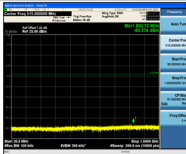
Band2-5MHz-QPSK-19175-1-0-Low-30-1000--60.57-PASS
