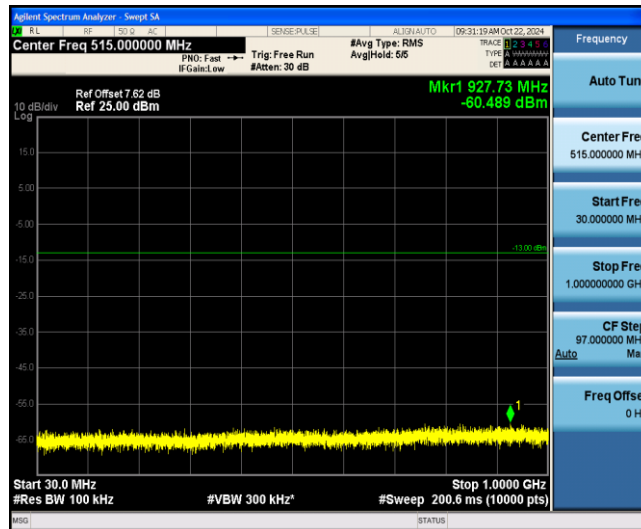
Band2-3MHz-QPSK-18615-1-0-Low-30-1000--60.49-PASS
