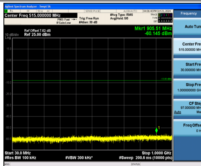
Band2-20MHz-QPSK-18700-1-0-Low-30-1000--60.15-PASS
