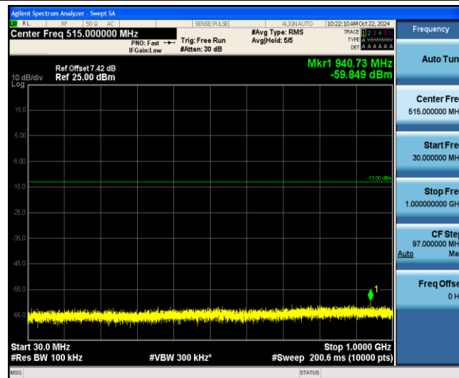
Band2-5MHz-16QAM-19175-1-0-Low-30-1000--59.85-PASS
