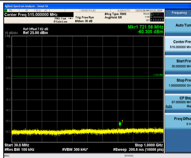
Band2-10MHz-QPSK-18900-1-0-Low-30-1000--60.31-PASS
