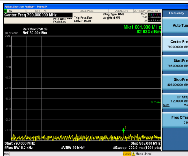
Band13-5MHz-QPSK-23255-1-0-Low-793-805--62.93-PASS
