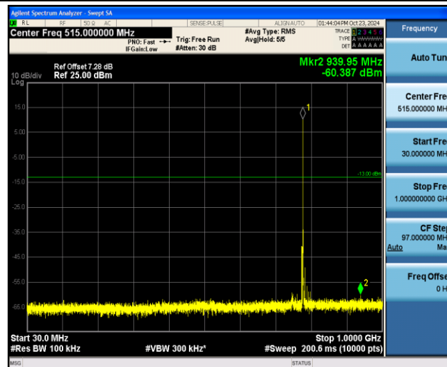
Band13-5MHz-QPSK-23255-1-0-Low-30-1000--60.39-PASS
