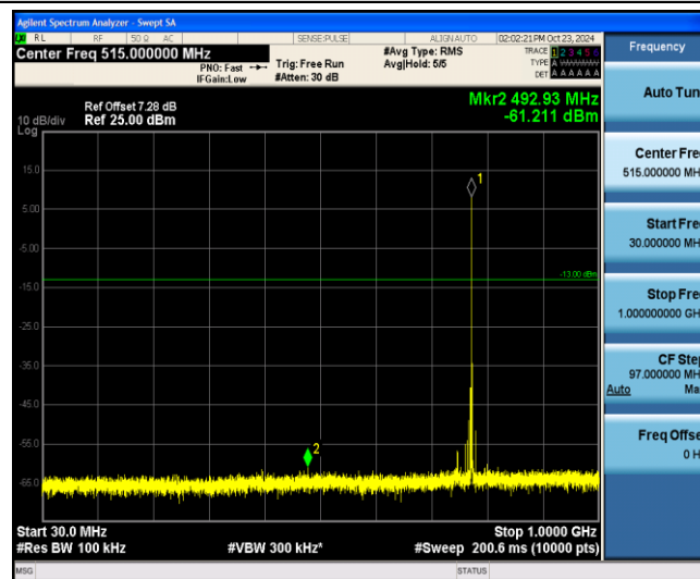
Band13-10MHz-16QAM-23230-1-0-Low-30-1000--61.21-PASS
