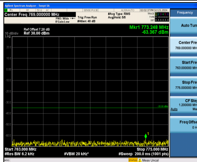
Band13-10MHz-16QAM-23230-1-0-Low-763-775--63.37-PASS
