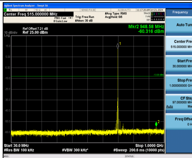
Band12-5MHz-QPSK-23095-1-0-Low-30-1000--60.32-PASS
