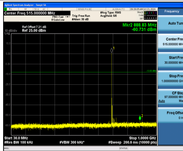
Band12-1.4MHz-QPSK-23017-1-0-Low-30-1000--60.73-PASS
