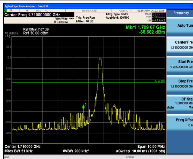
Band4-10MHz-QPSK-20000-1-0-Low--38.68-PASS
