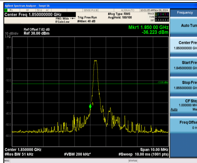
Band25-5MHz-QPSK-26065-1-0-Low--36.22-PASS
