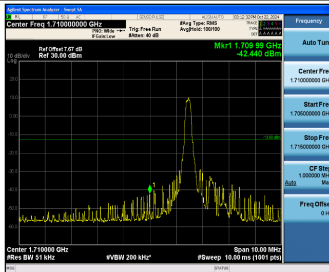
Band4-20MHz-QPSK-20050-1-0-Low--42.44-PASS
