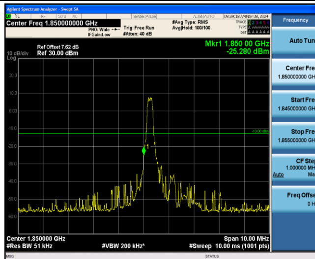
Band25-1.4MHz-QPSK-26047-1-0-Low--25.28-PASS
