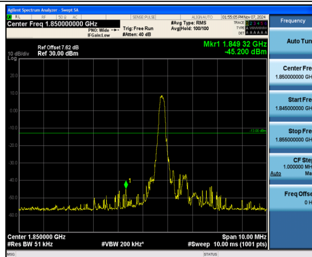
Band25-10MHz-QPSK-26090-1-0-Low--45.20-PASS
