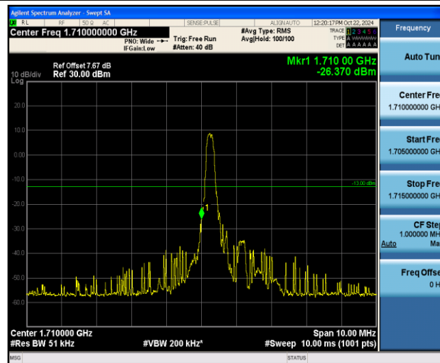
Band4-1.4MHz-16QAM-19957-1-0-Low--26.37-PASS
