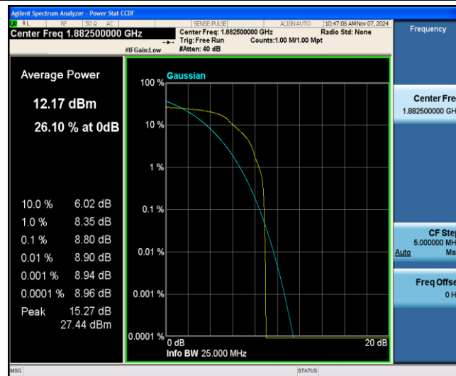
Band25-1.4MHz-QPSK-26365-1-0-Low-8.80-&lt;=13-PASS
