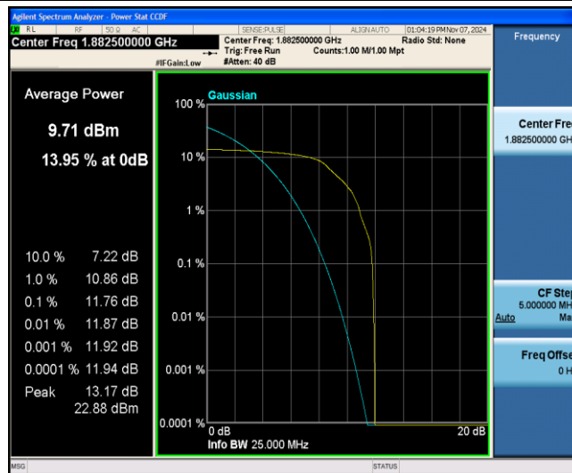
Band25-3MHz-QPSK-26365-1-0-Low-11.76-&lt;=13-PASS
