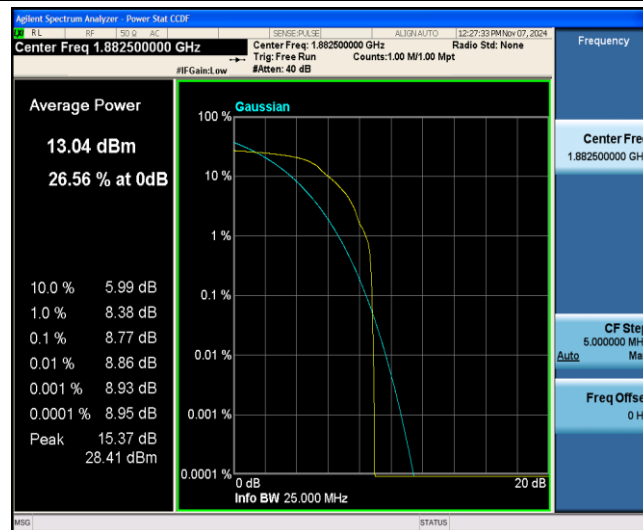
Band25-5MHz-QPSK-26365-1-0-Low-8.77-&lt;=13-PASS
