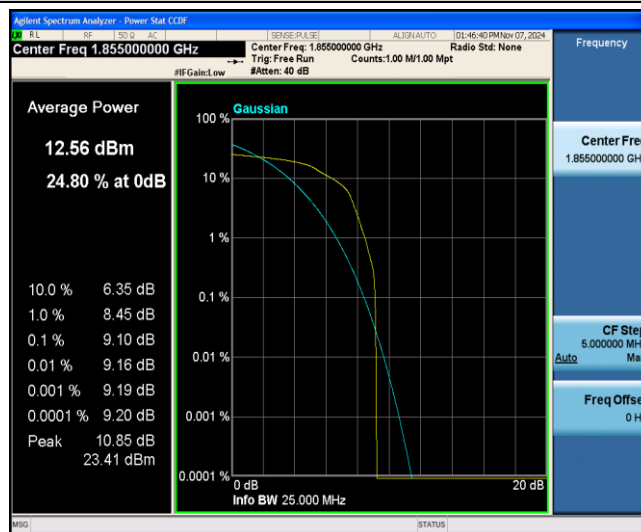
Band25-10MHz-16QAM-26090-1-0-Low-9.10-&lt;=13-PASS
