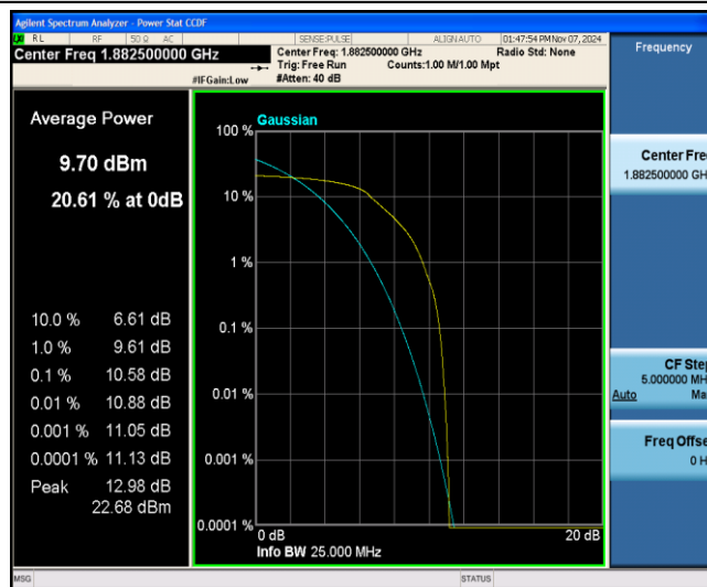
Band25-10MHz-QPSK-26365-6-0-Low-10.58-&lt;=13-PASS
