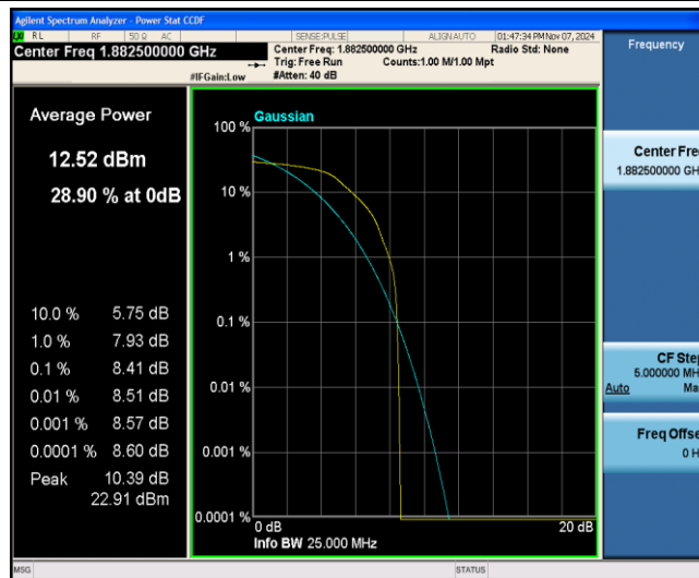
Band25-10MHz-QPSK-26365-1-0-Low-8.41-&lt;=13-PASS
