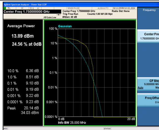
Band4-10MHz-16QAM-20350-1-0-Low-9.10-=&lt;=13-PASS
