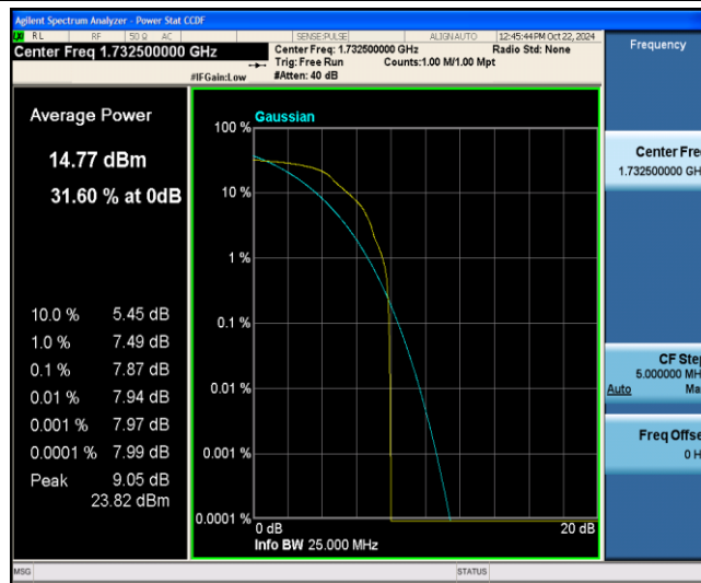
Band4-3MHz-QPSK-20175-1-0-Low-7.87-&lt;=13-PASS
