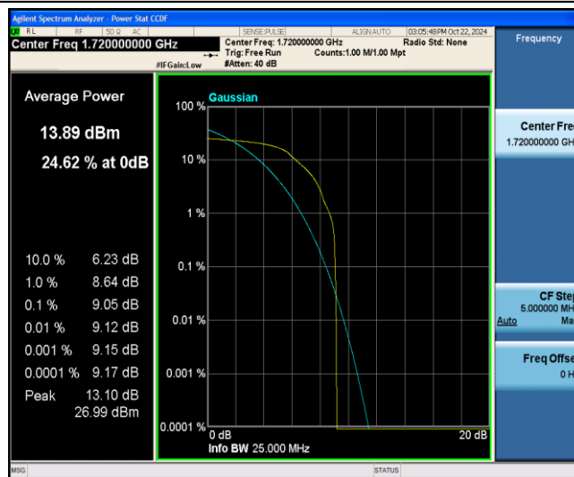
Band4-20MHz-QPSK-20050-1-0-Low-9.05-&lt;=13-PASS
