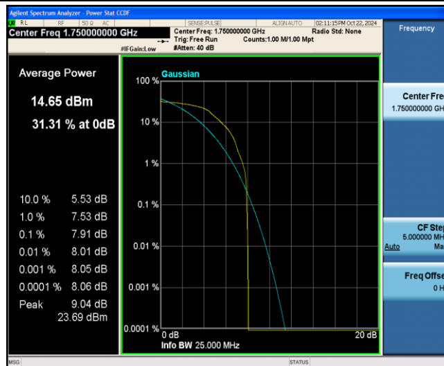
Band4-10MHz-QPSK-20350-1-0-Low-7.91-&lt;=13-PASS
