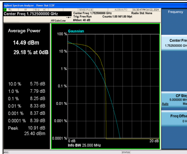
Band4-5MHz-QPSK-20375-1-0-Low-8.25-&lt;=13-PASS
