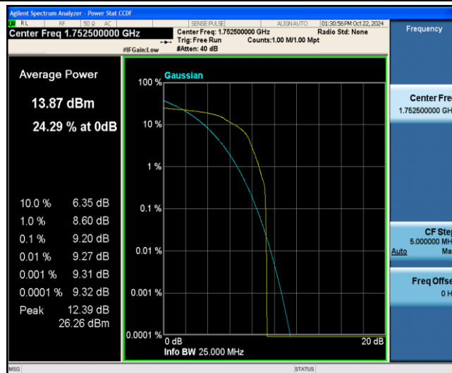
Band4-5MHz-16QAM-20375-1-0-Low-9.20-&lt;=13-PASS
