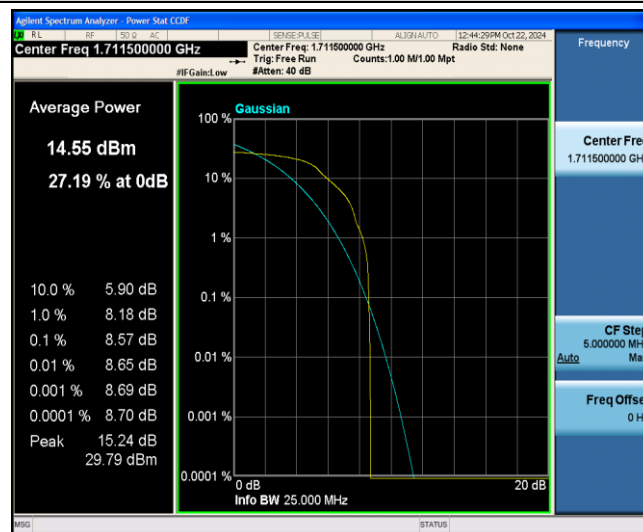
Band4-3MHz-QPSK-19965-1-0-Low-8.57-&lt;=13-PASS
