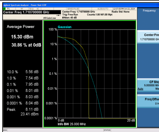
Band4-1.4MHz-QPSK-19957-1-0-Low-7.95-≤13-PASS
