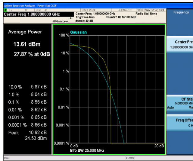
Band2-5MHz-QPSK-18900-1-0-Low-8.55-&lt;=13-PASS
