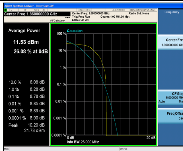
Band2-20MHz-QPSK-18700-1-0-Low-8.78-&lt;=13-PASS
