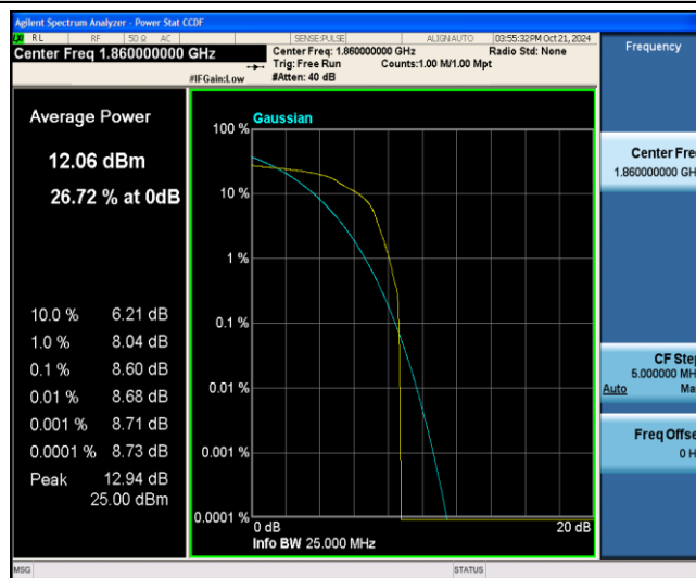
Band2-20MHz-16QAM-18700-1-0-Low-8.60-&lt;=13-PASS
