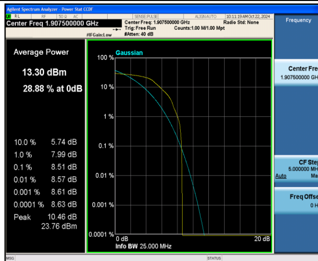
Band2-5MHz-QPSK-19175-1-0-Low-8.51-&lt;=13-PASS
