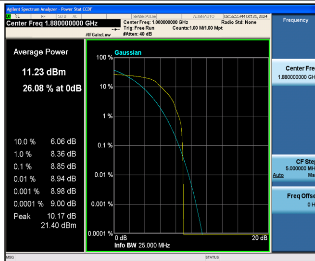
Band2-20MHz-QPSK-18900-1-0-Low-8.85-&lt;=13-PASS
