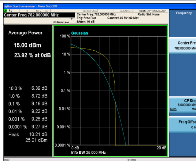
Band13-5MHz-16QAM-23230-1-0-Low-9.16-13-PASS
