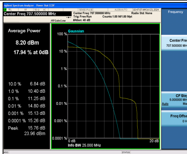
Band12-5MHz-QPSK-23095-1-0-Low-11.25-&lt;=13-PASS
