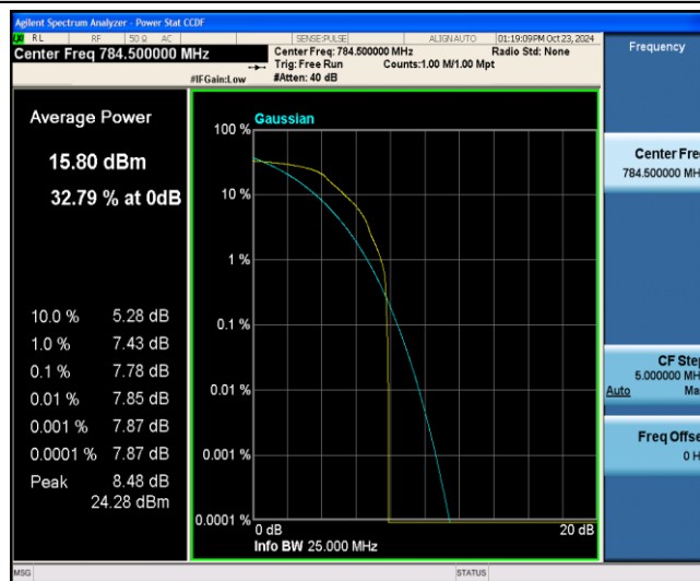
Band13-5MHz-QPSK-23255-1-0-Low-7.78-&lt;=13-PASS
