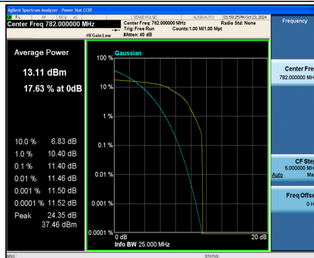
Band13-10MHz-16QAM-23230-1-0-Low-11.40-=&lt;=13-PASS
