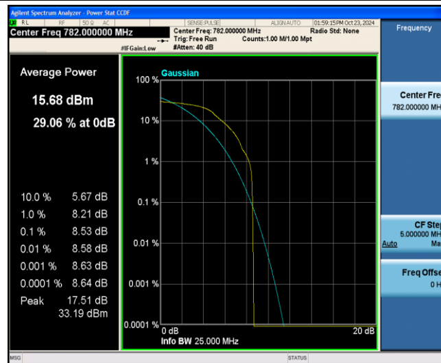
Band13-10MHz-QPSK-23230-1-0-Low-8.53-=&lt;=13-PASS
