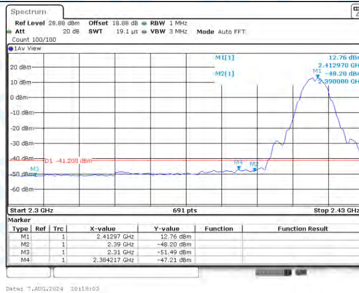
11B_Ant1_Low_2412_AV
