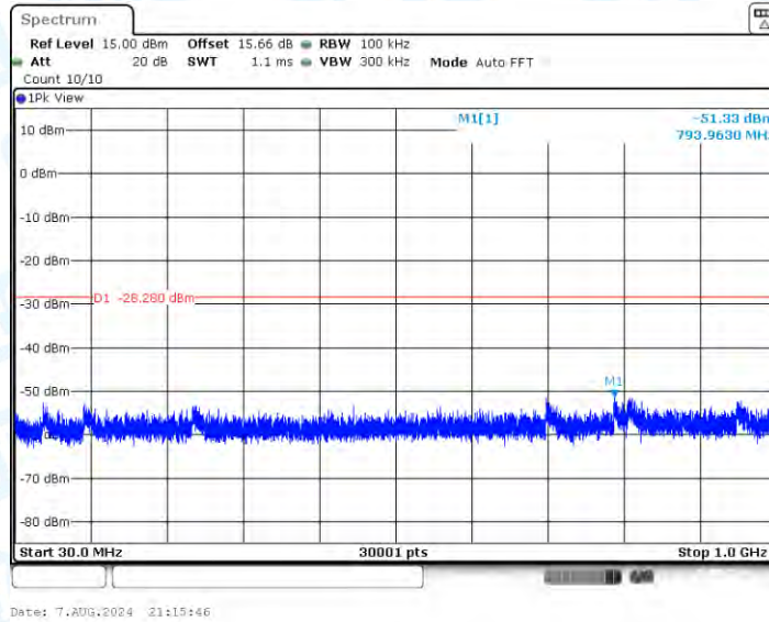
11AX20SISO_Ant1_2412_30~1000
