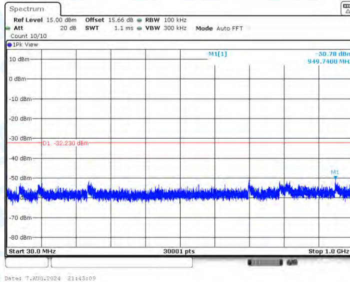
11AX40SISO_Ant1_2437_30~1000
