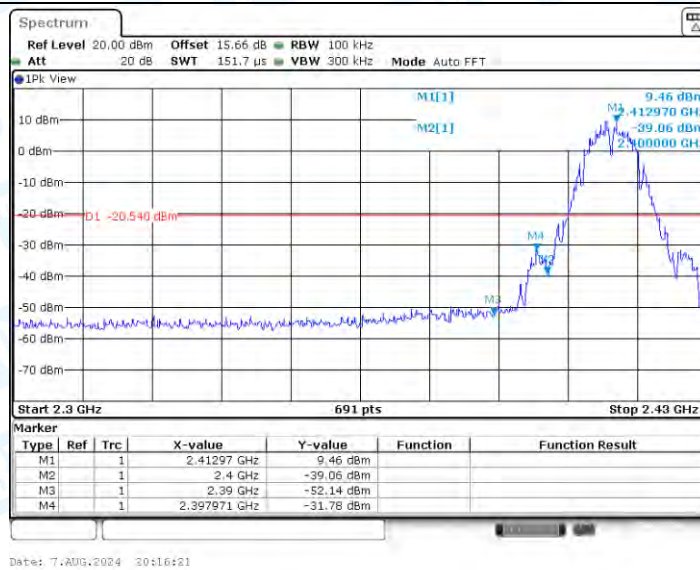
11B_Ant1_Low_2412
