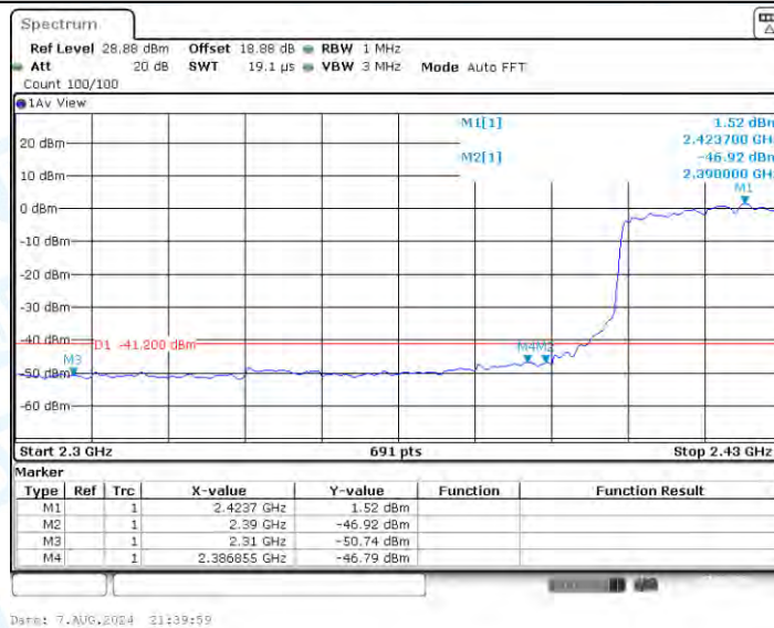
11AX40SISO_Ant1_Low_2422_AV
